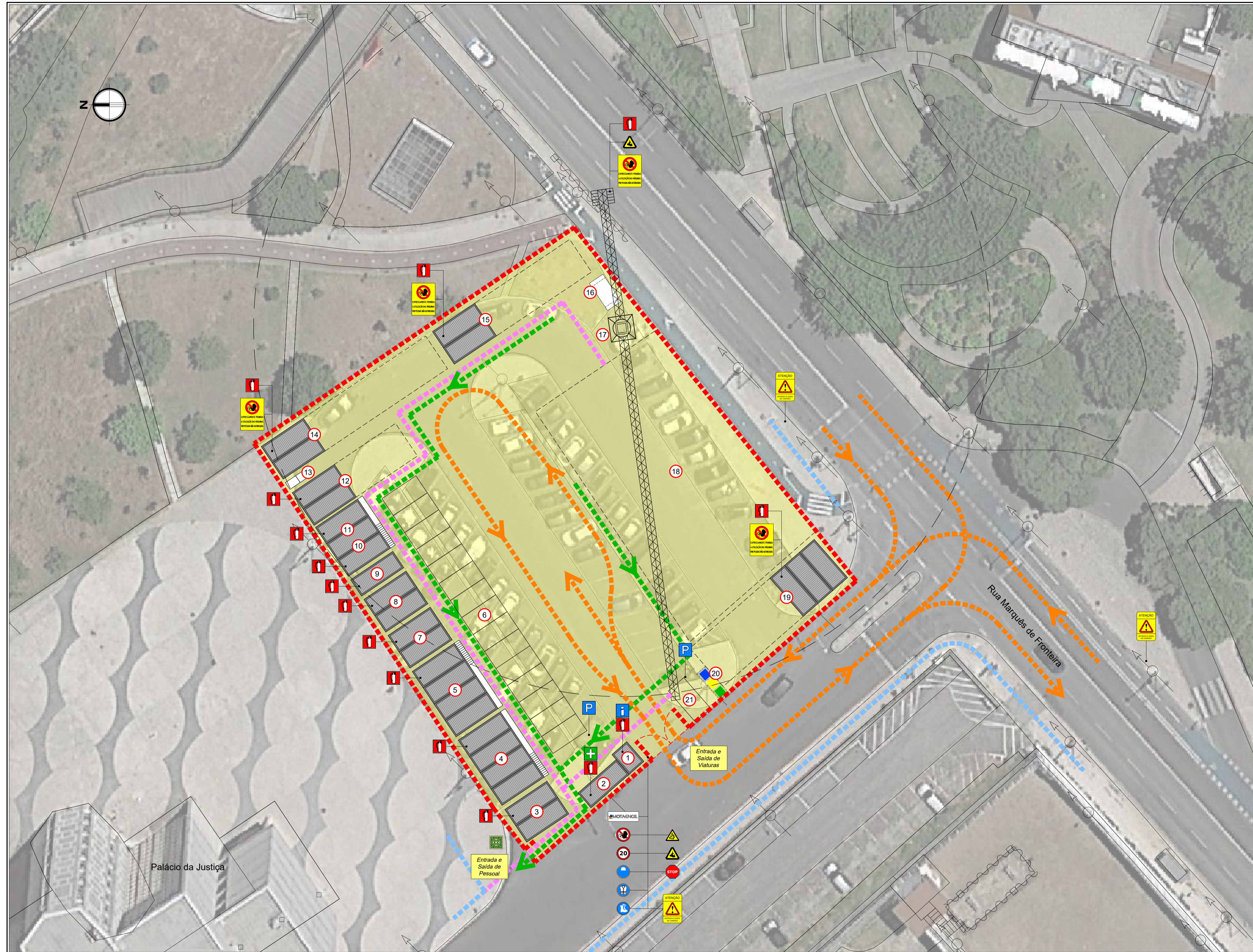
Estaleiro Central (Estacionamento Palácio da Justiça) - Planta de Estaleiro e Sinalização de Segurança A1 - Escala 1:250
