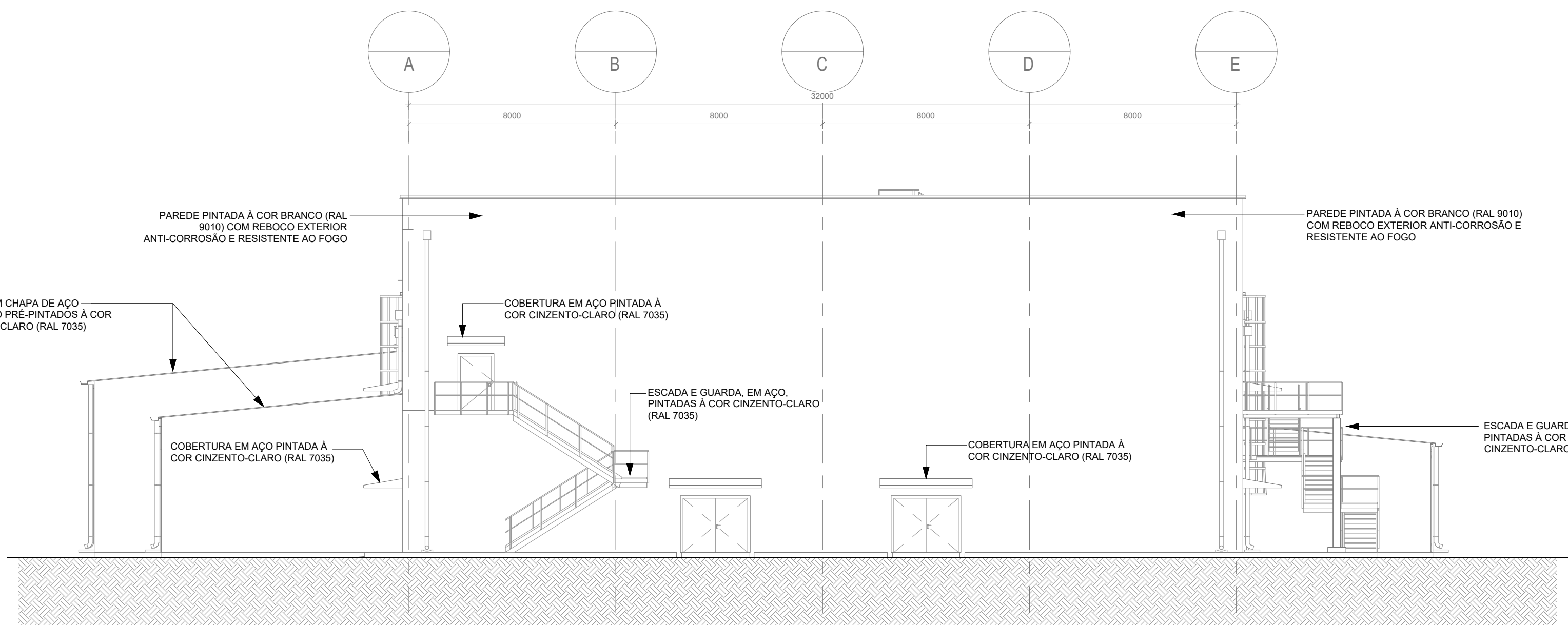
ALÇADO NORTE
