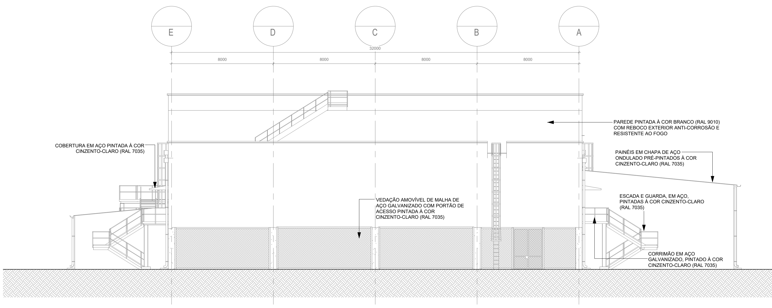
ALÇADO SUL
