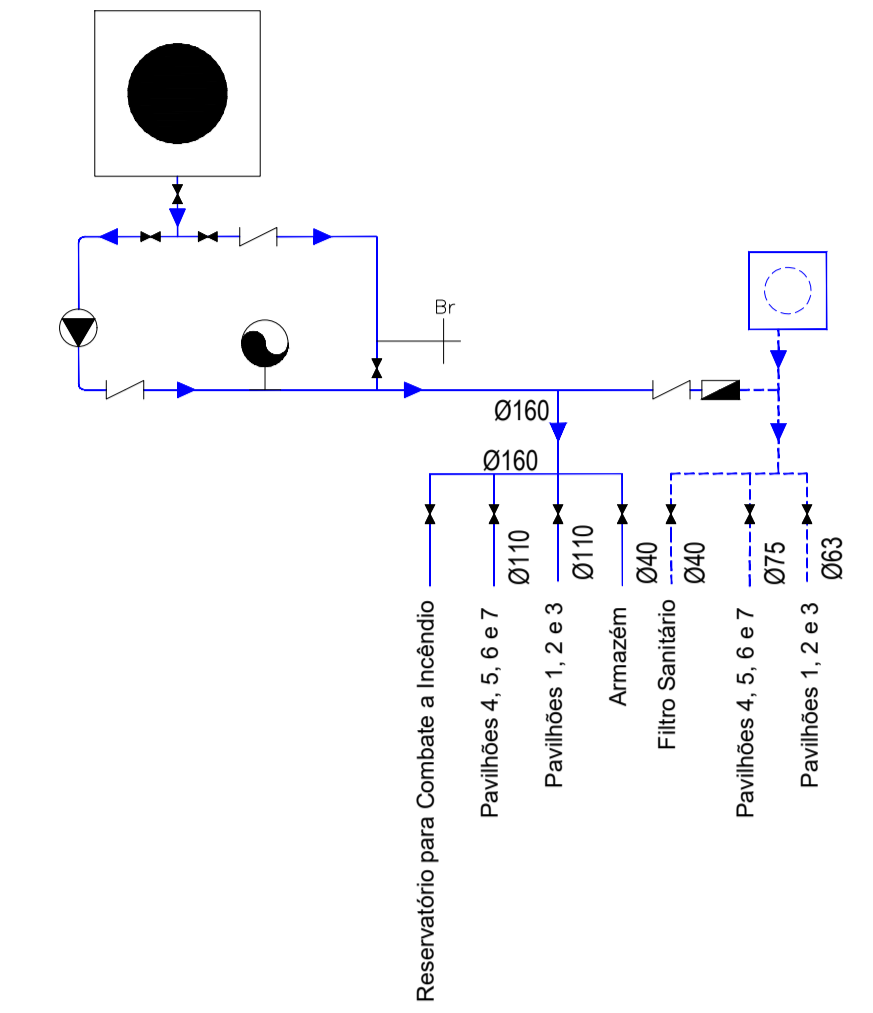
ESQUEMA DO SISTEMA DE BOMBAGEM E DESINFECÇÃO DA ÁGUA RESERVATÓRIO 1
