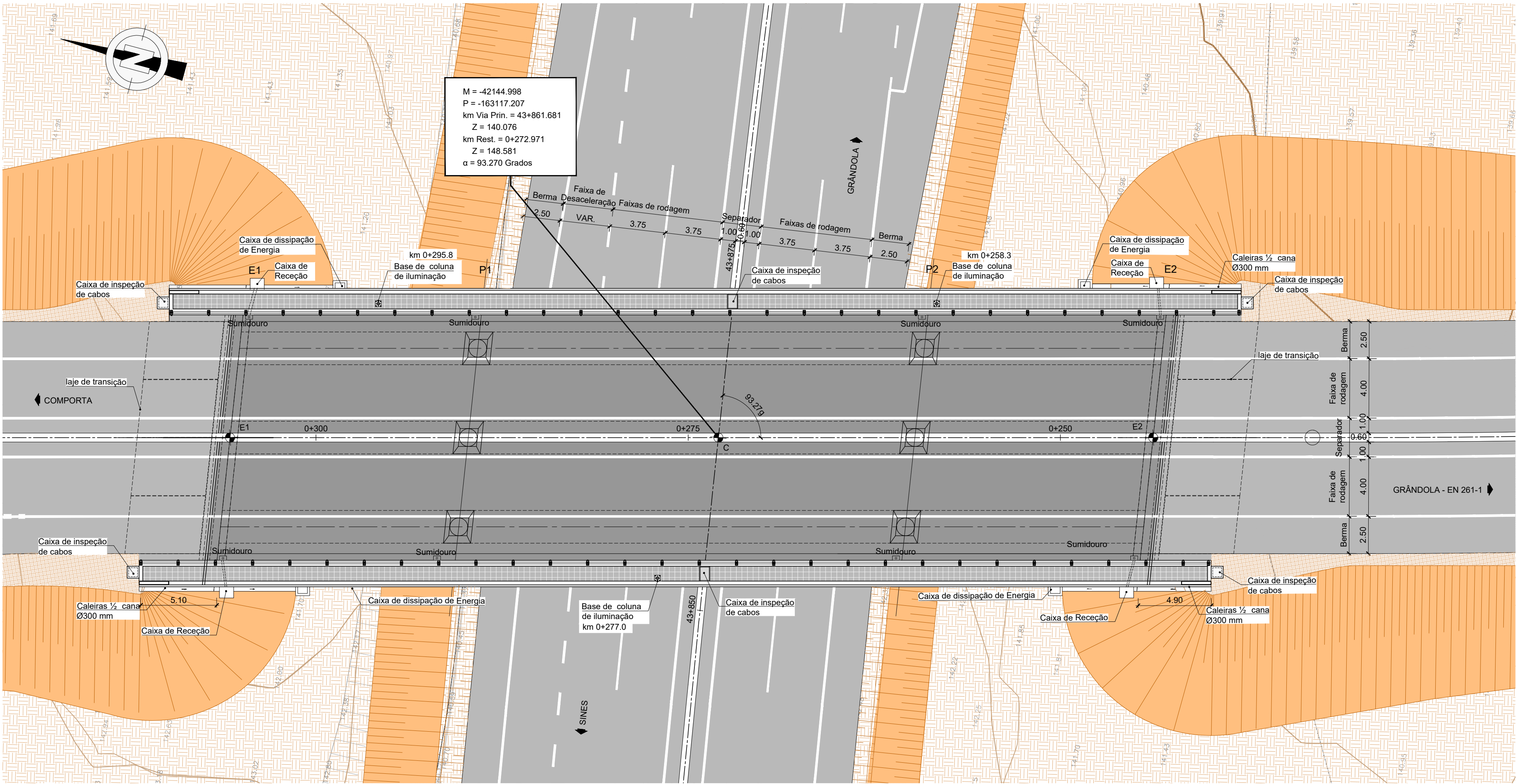
PLANTA ESC.=1:200
