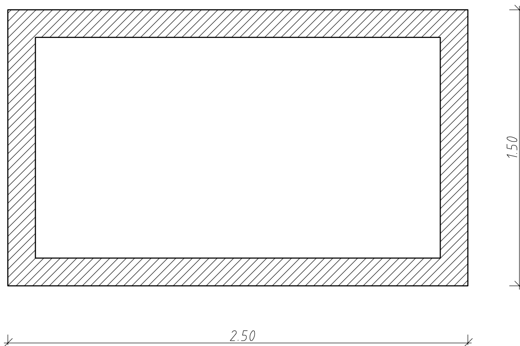
PLANTA - FOSSA
