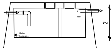
FOSSA SÉPTICA
