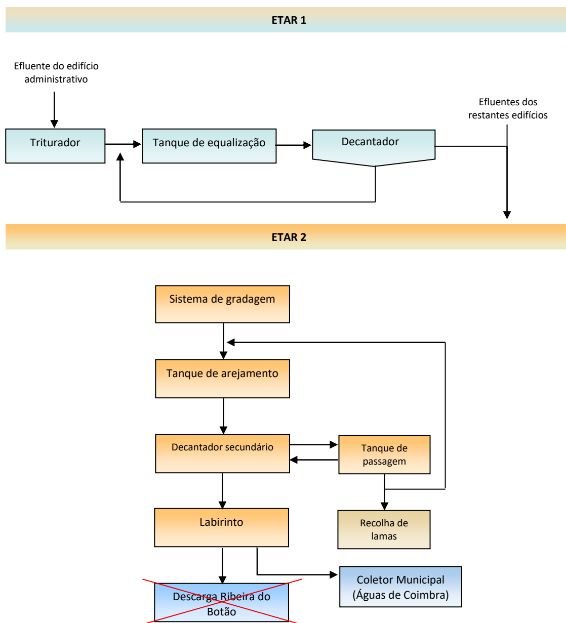
Figura 1 – Fluxograma da ETAR de águas residuais domésticas do Centro de Produção de Souselas (LT1)
