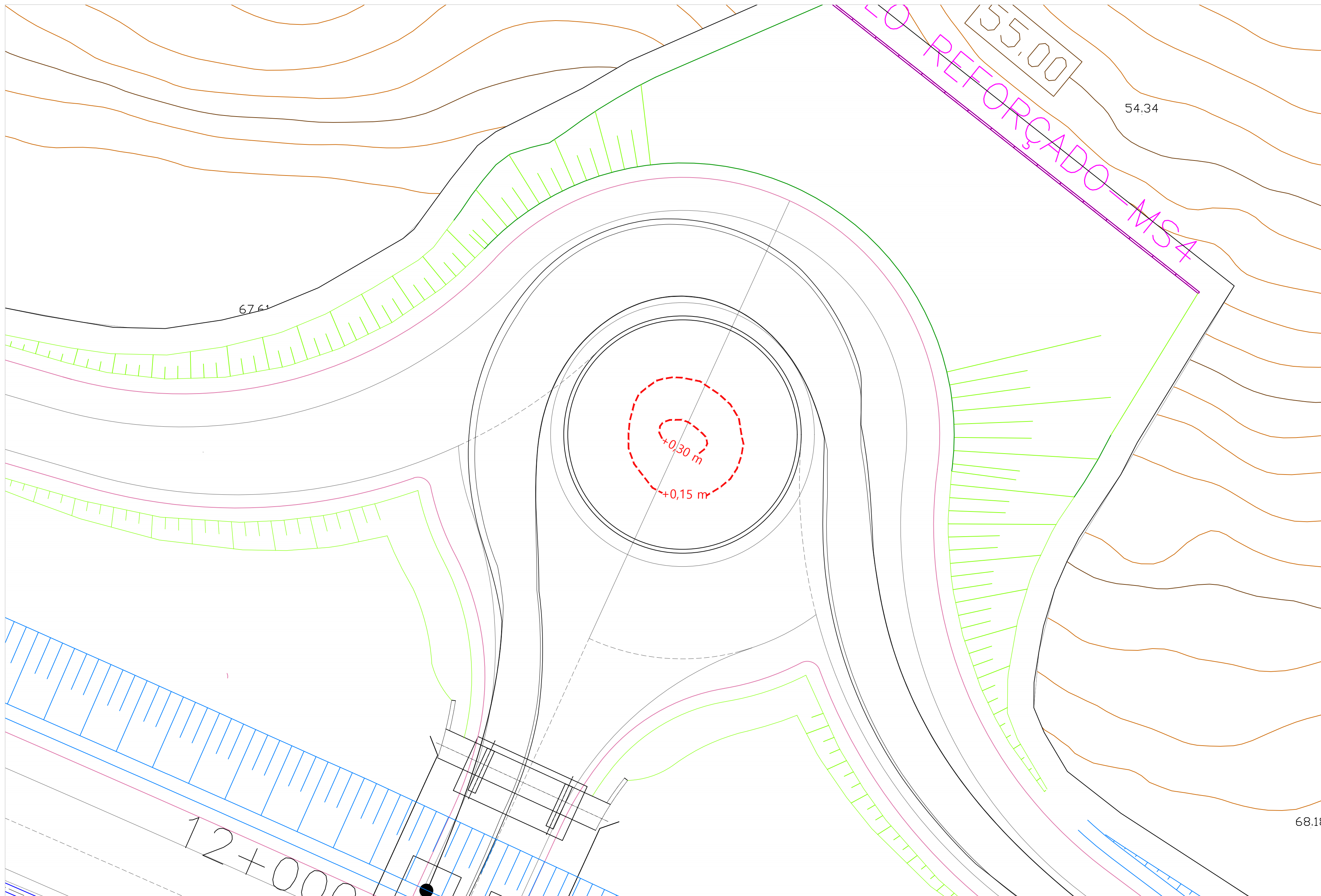
ROTUNDA DE LIGAÇÃO A TRAVASSÔ - MODELAÇÃO
