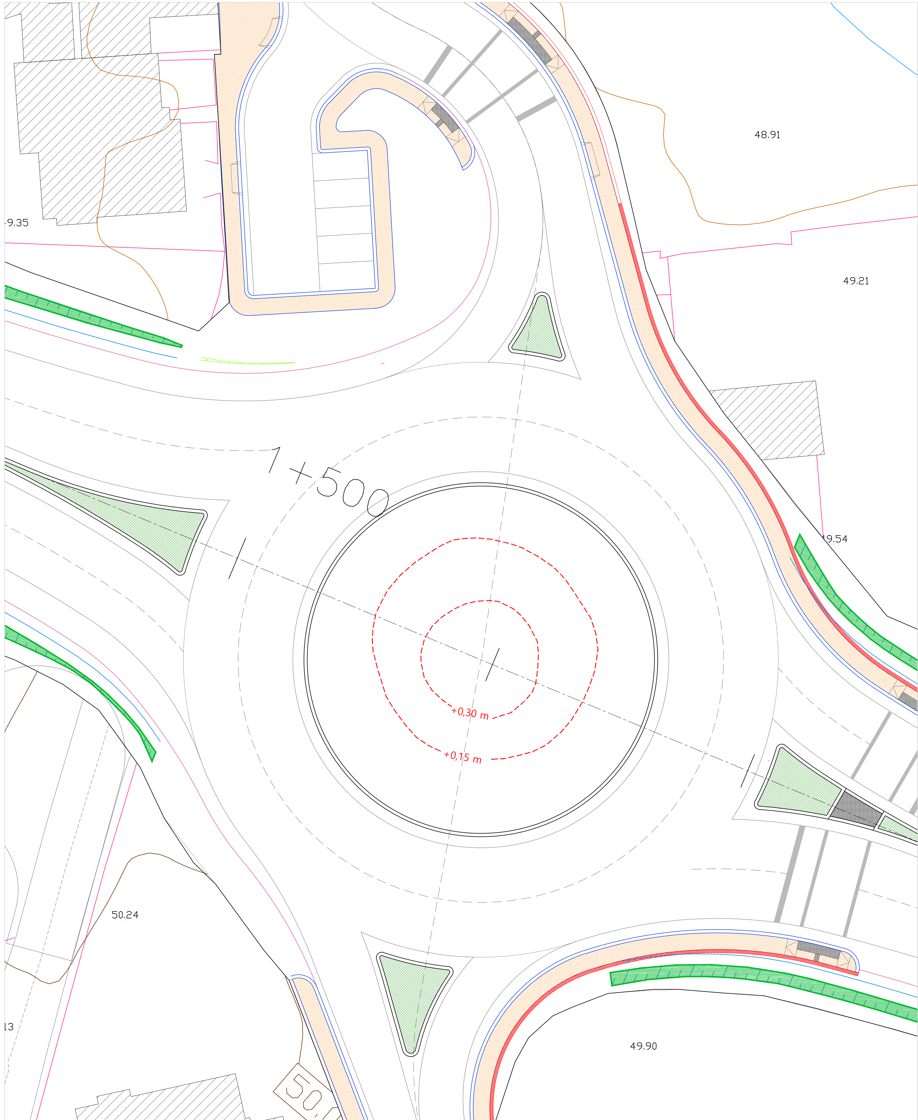
ROTUNDA DE CAMPINOS - Modelação
