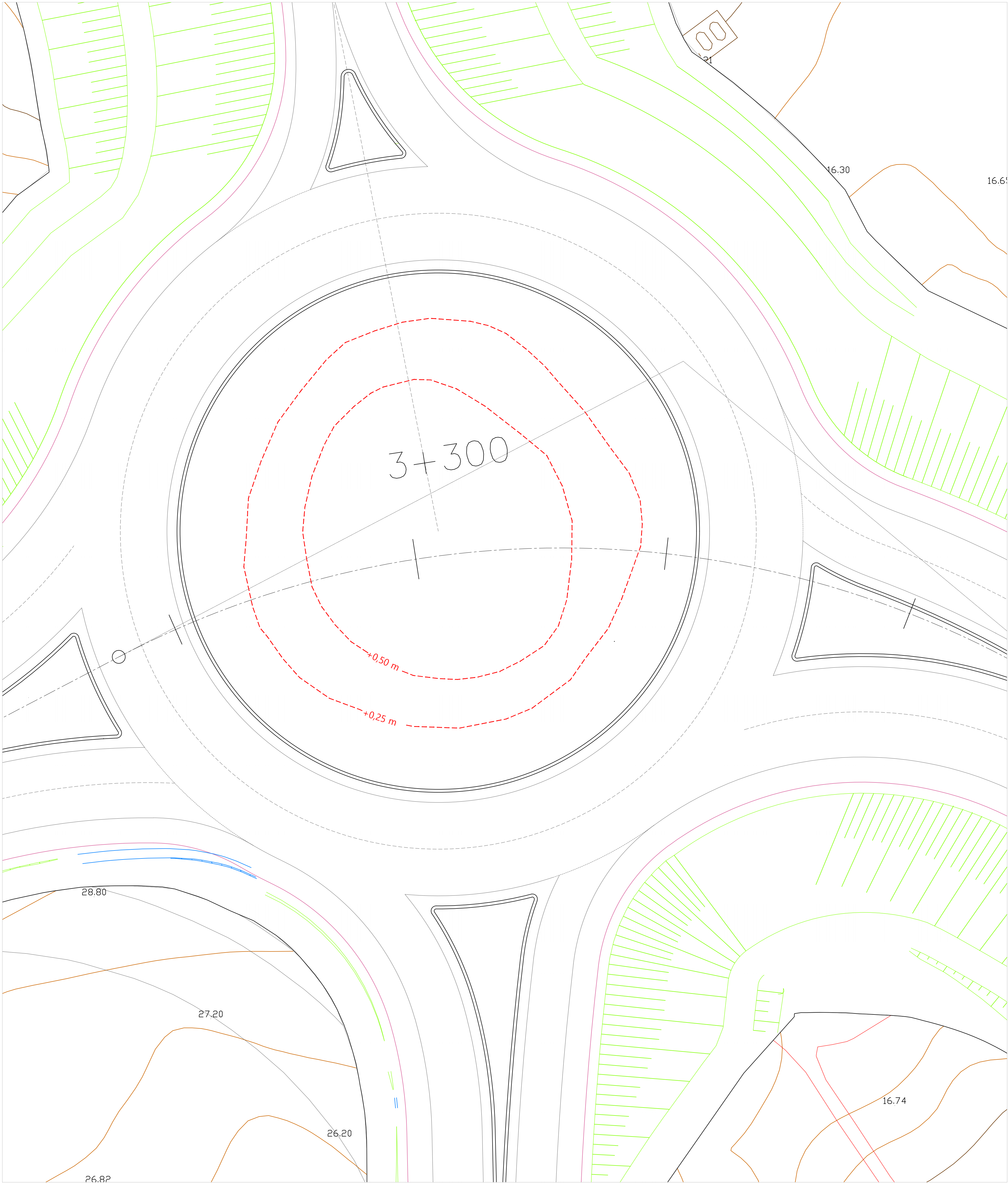
ROTUNDA DE AZENHAS - MODELAÇÃO
