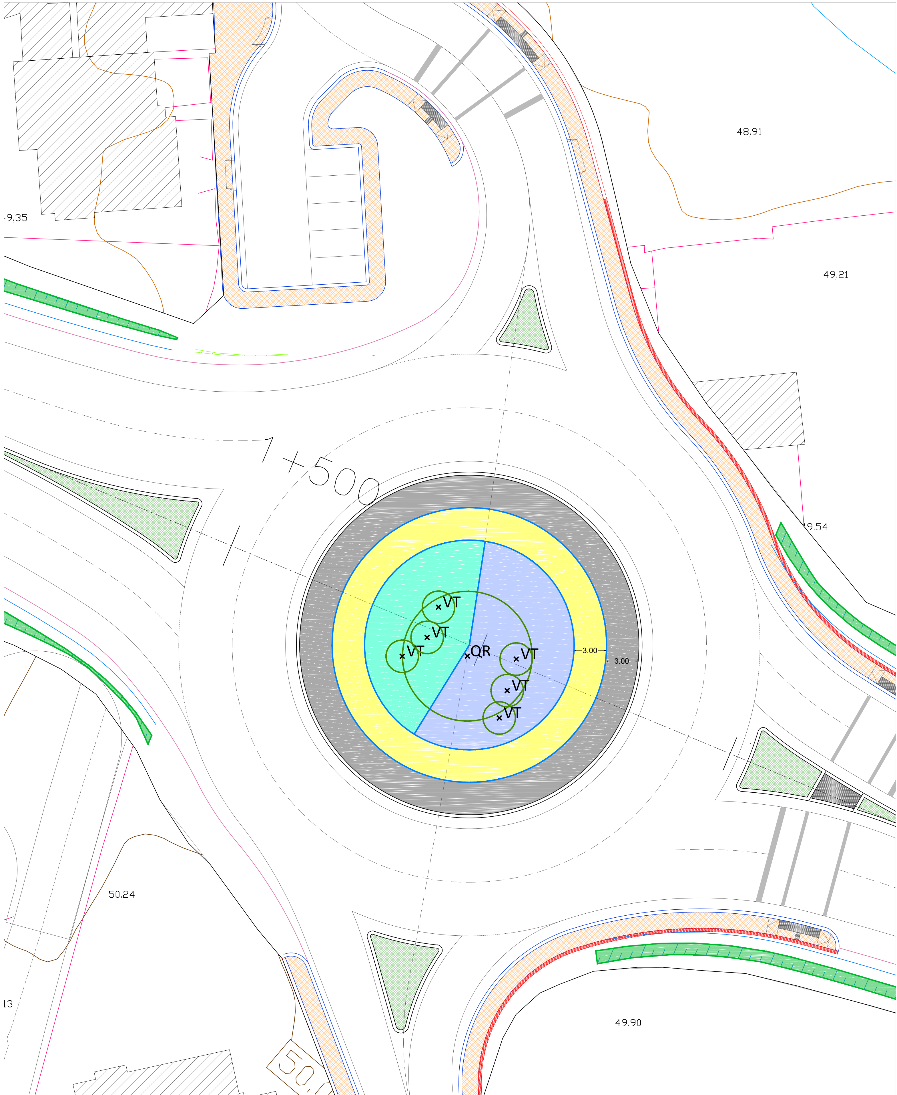
ROTUNDA DE CAMPINOS
