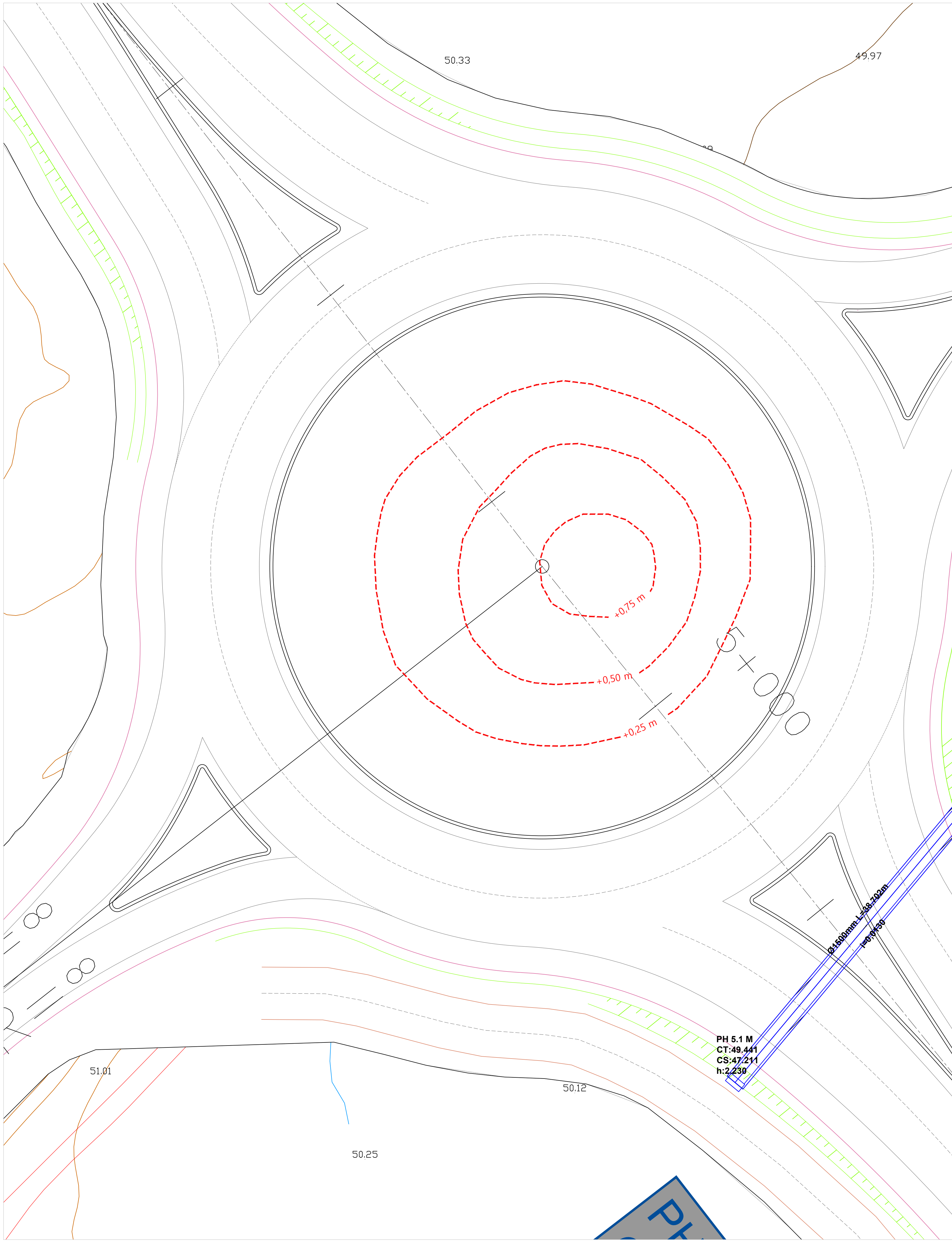
ROTUNDA DE EIXO - MODELAÇÃO
