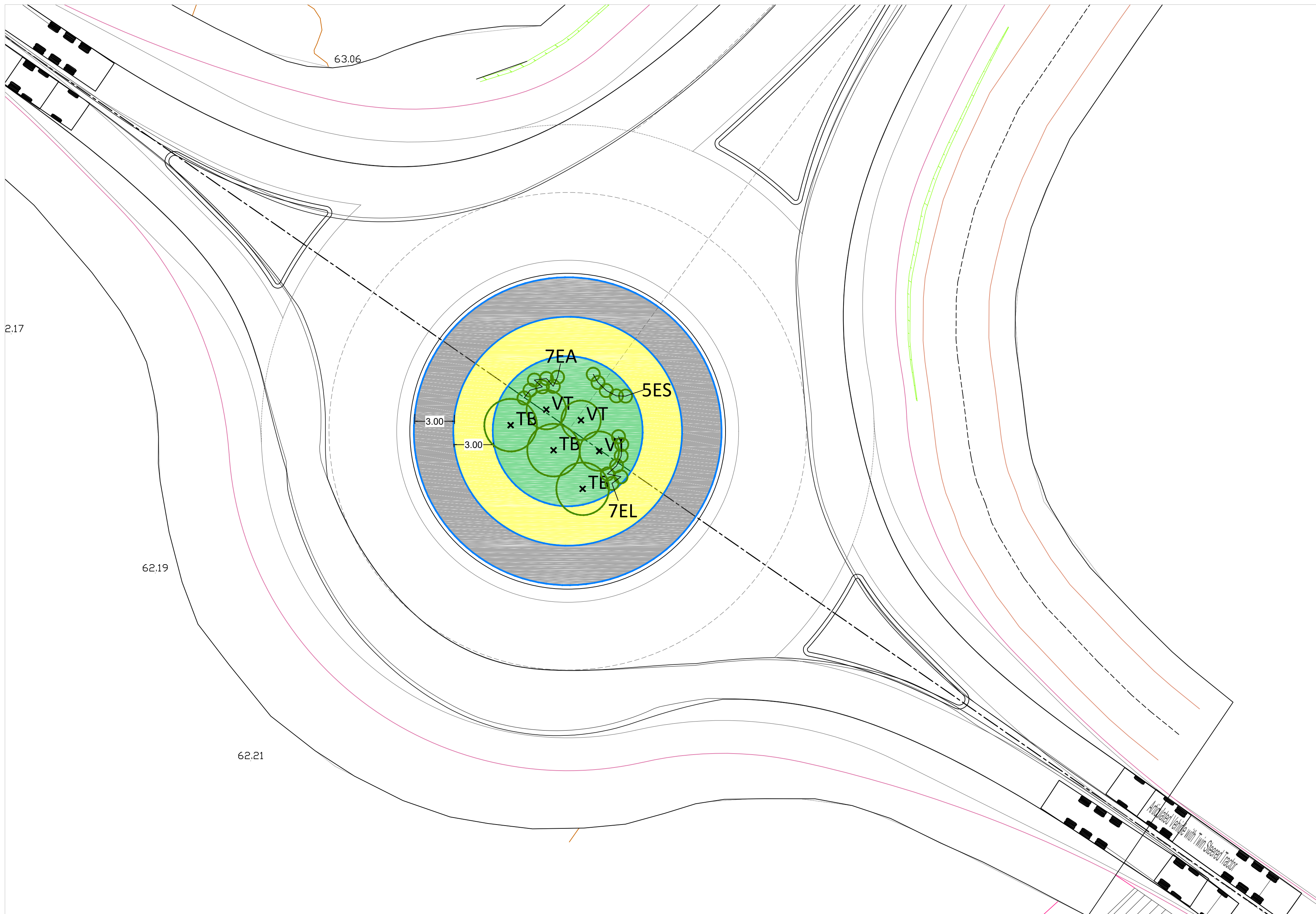
ROTUNDA DE TRAVASSÔ
