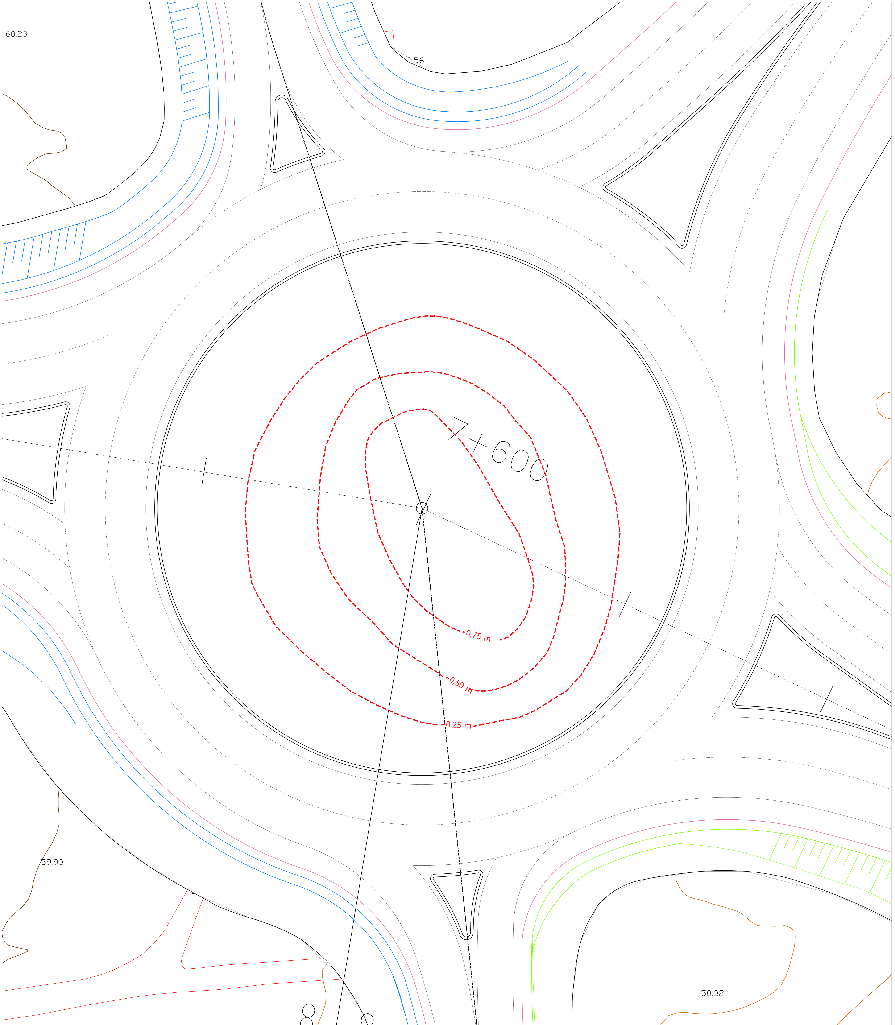
ROTUNDA DE EIROL - MODELAÇÃO
