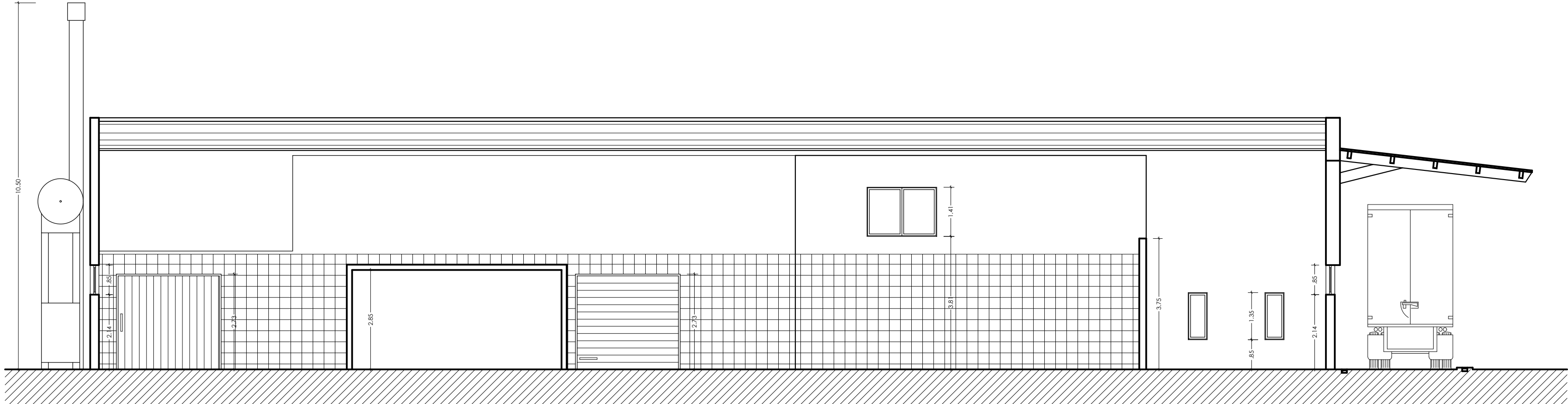
CORTE CD
