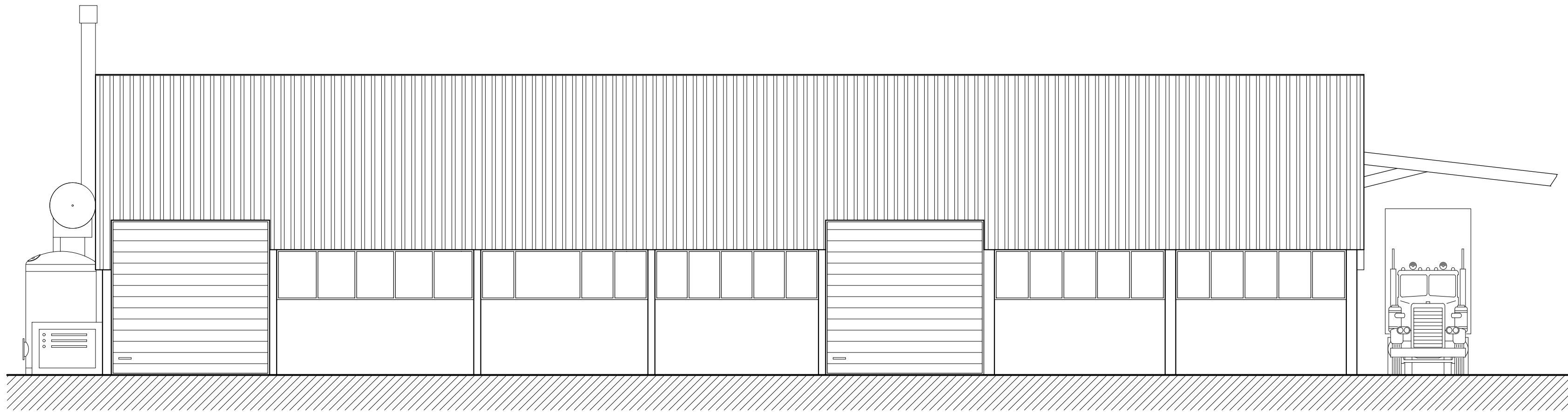
ALÇADO TARDOZ
