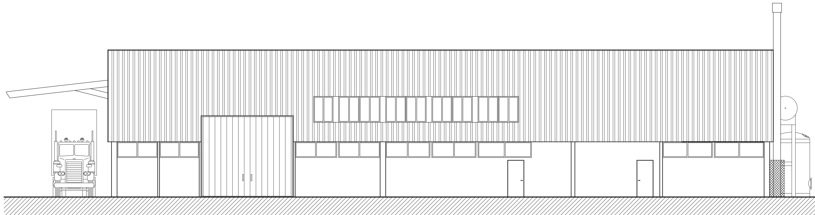
ALÇADO PRINCIPAL
