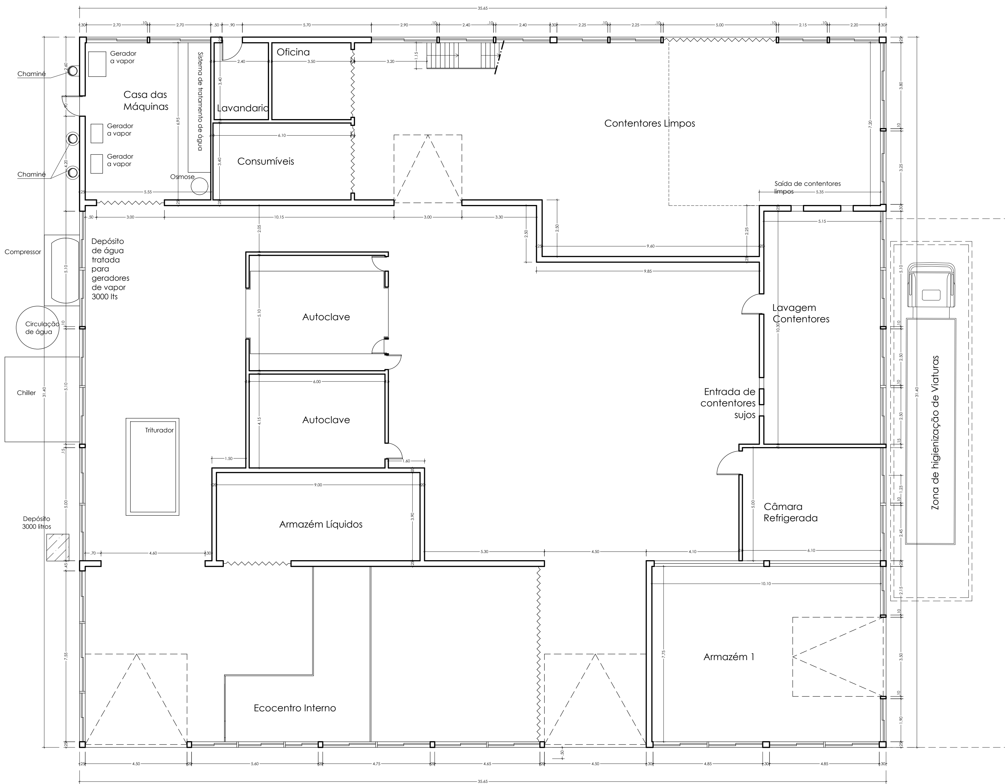
PLANTA DO PISO 0
