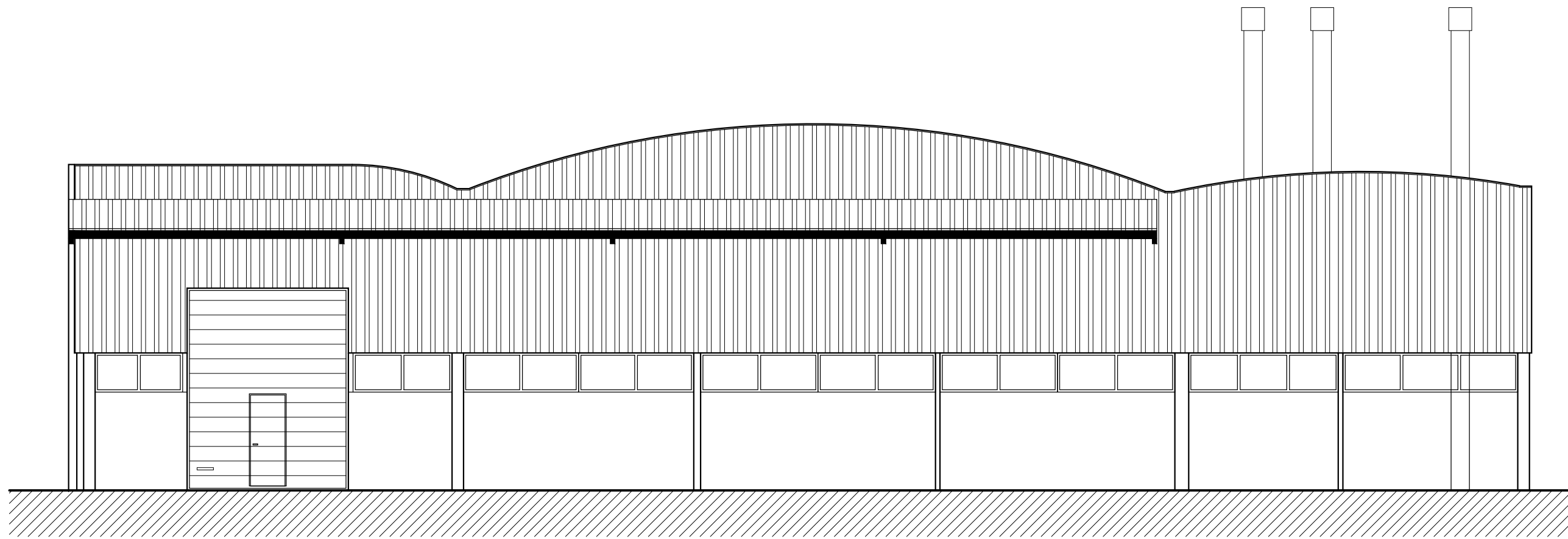
ALÇADO LATERAL ESQUERDO
