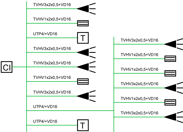
DIAGRAMA DE CABOS E LIGAÇÕES
