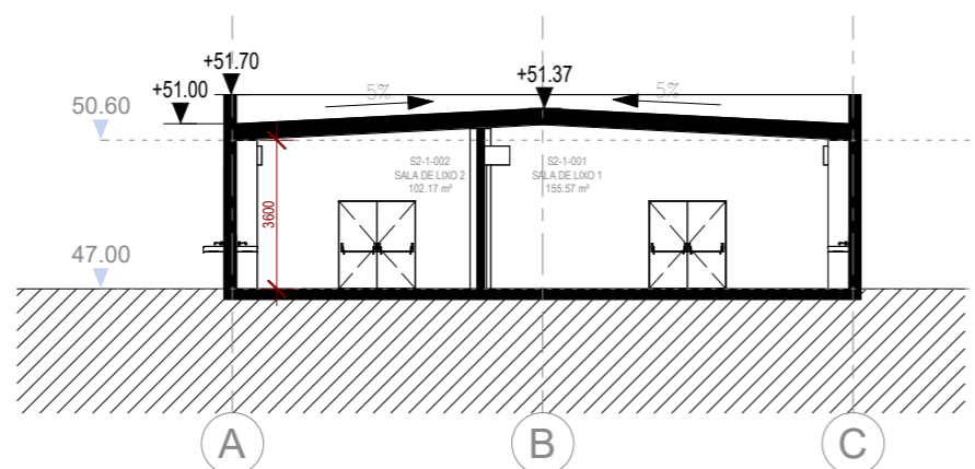
CORTE / SECTION B 1 : 200
