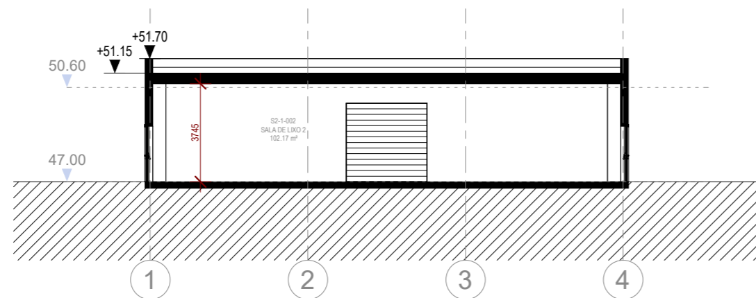
CORTE / SECTION A 1 : 200
