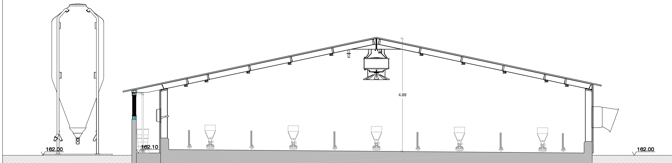
CORTE 07
