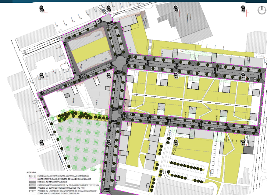
Planta do loteamento com a rede viária, identificando estacionamento e materiais das diferentes vias.
