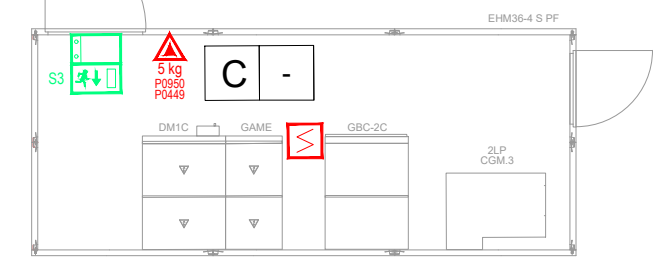
PLANTA POSTO DE SECCIONAMENTO
