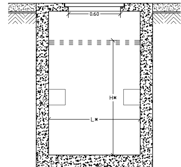
CORTE C-C
