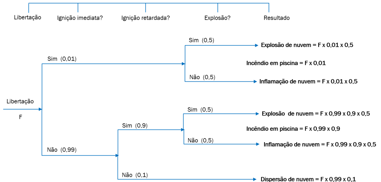
Figura 4- Árvore de evento tipo 4 - Libertações instantâneas de gasóleo
