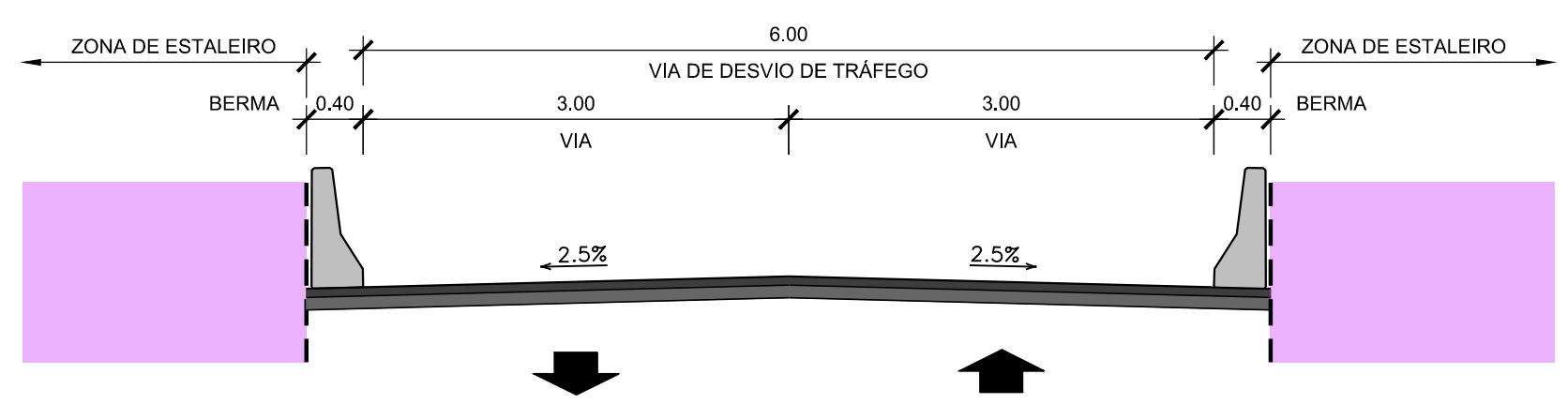
SECÇÃO A-A' ESC. 1:50
