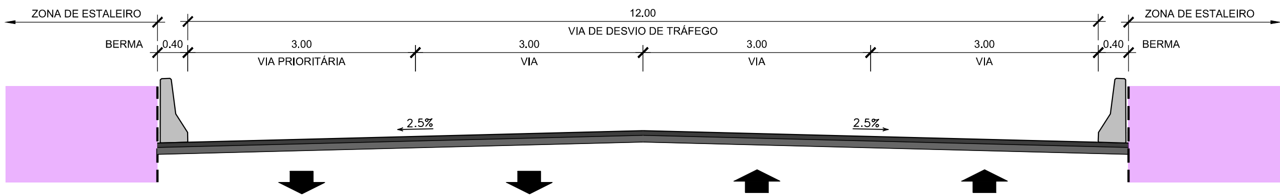
SECÇÃO A-A' ESC. 1:50
