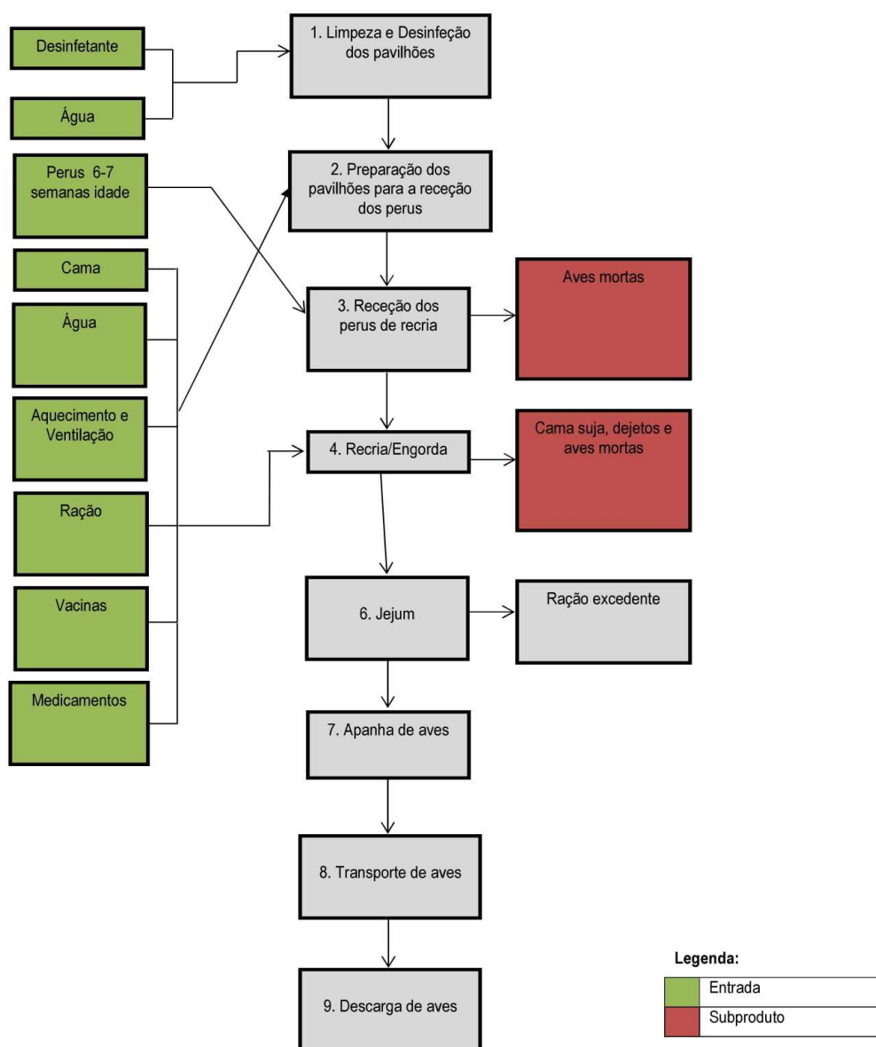
FIGURA 1. FLUXOGRAMA DE PRODUÇÃO
