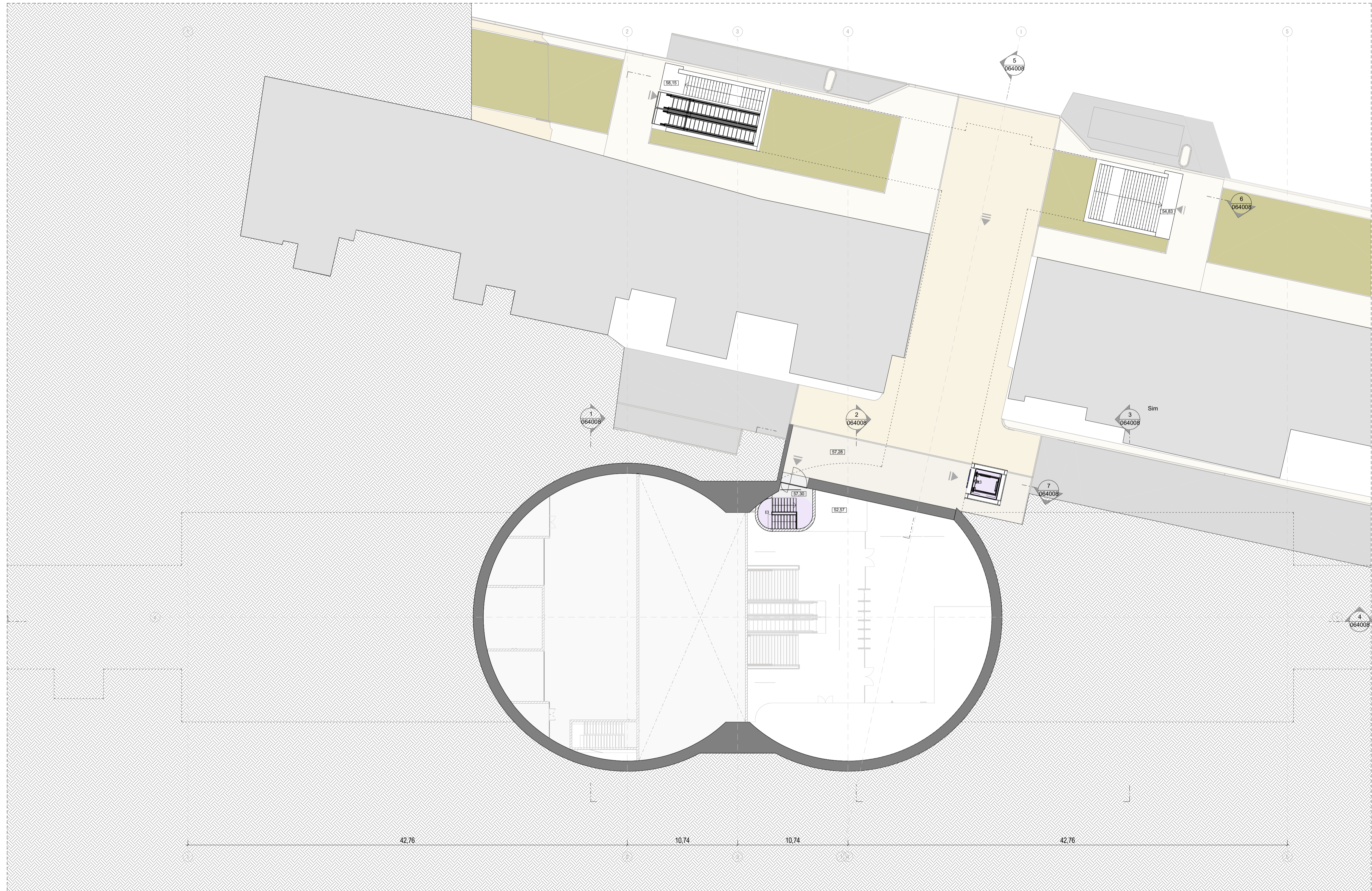
PLANTA DO ACESSO 3 1 : 200
