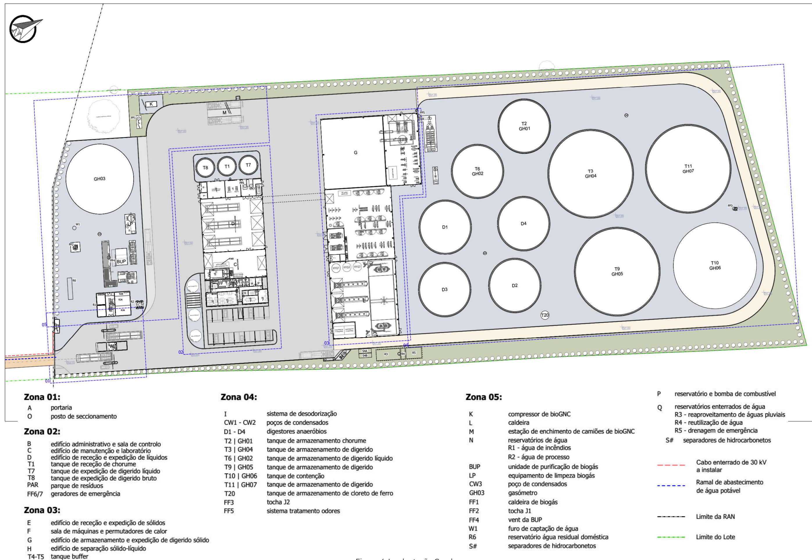
Figura 4. Implantação Geral
