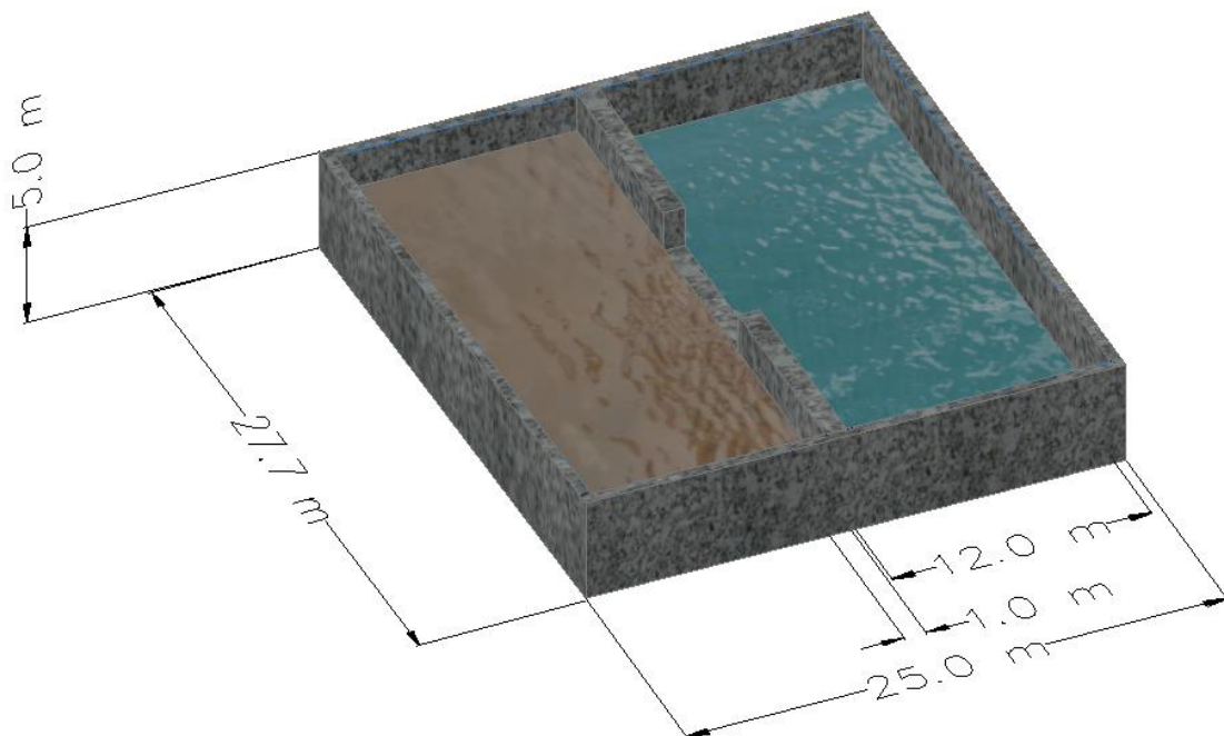
Figura 4 - Modelação da charca existente.
