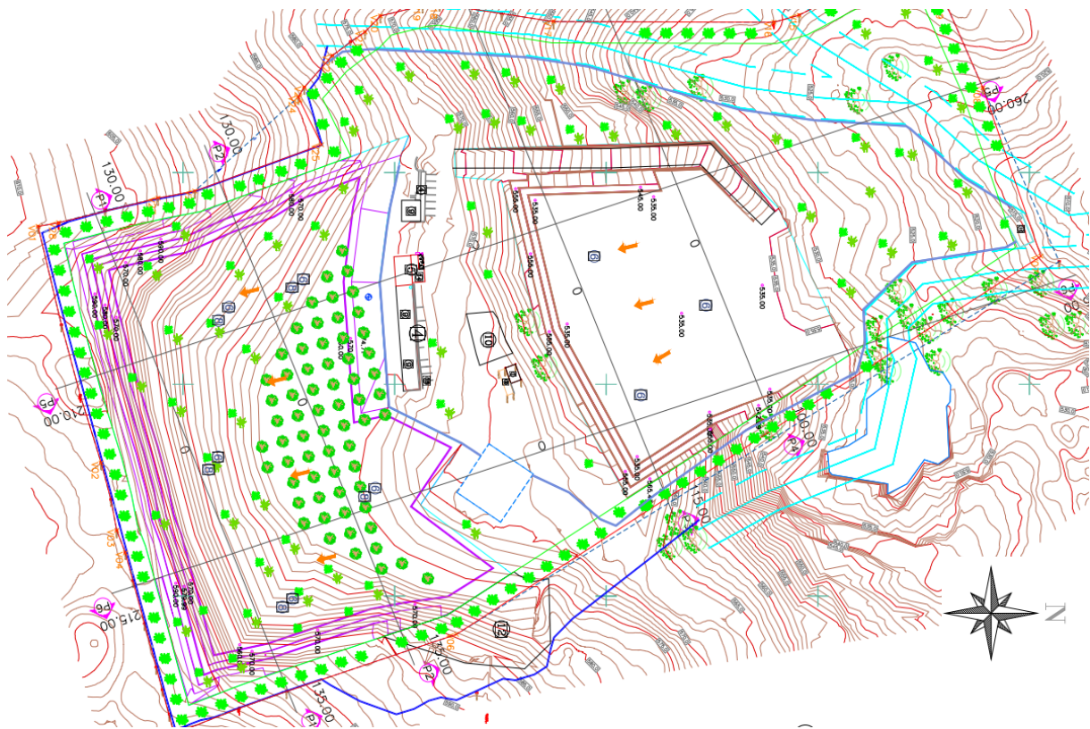
Figura 1 - Planta de Escavação Final
