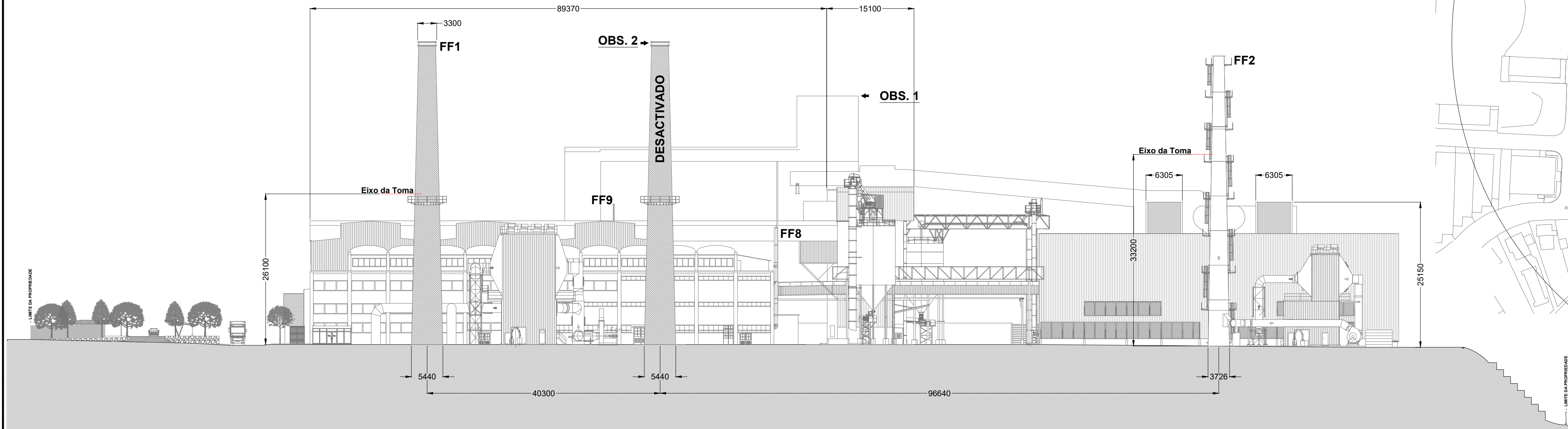
* Alçado Sul *
