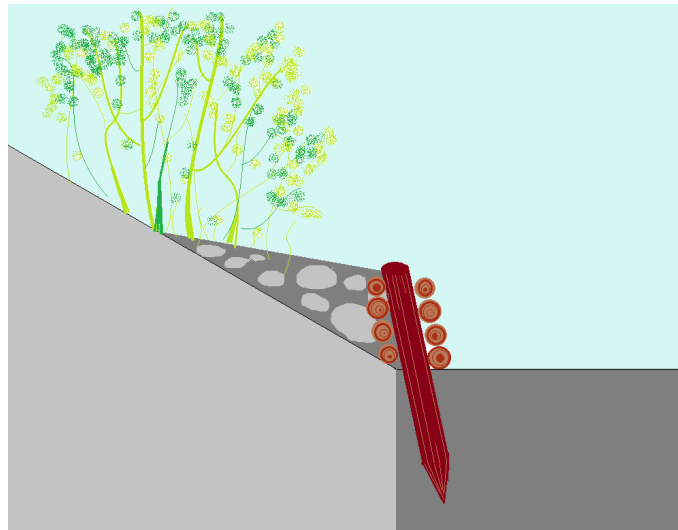
Figura 6.2 – Técnica de Bioengenharia: Entrançado.
