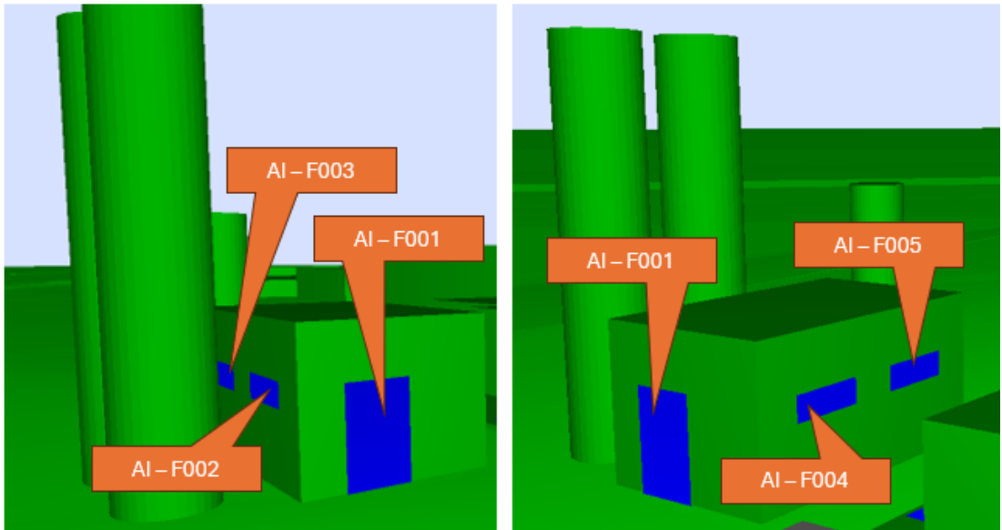
Ilustração 12. Envolventes no Edifício de Espessamento e Desidratação de Lamas
