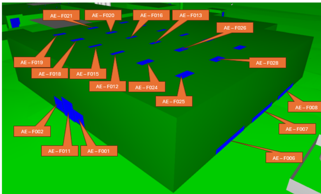
Ilustração 20. Envolventes no Edifício de Osmose Inversa
