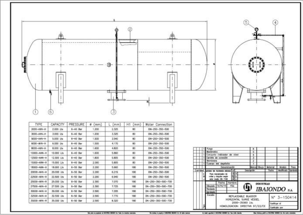
Conjunto antiariete horizontal con membrana
