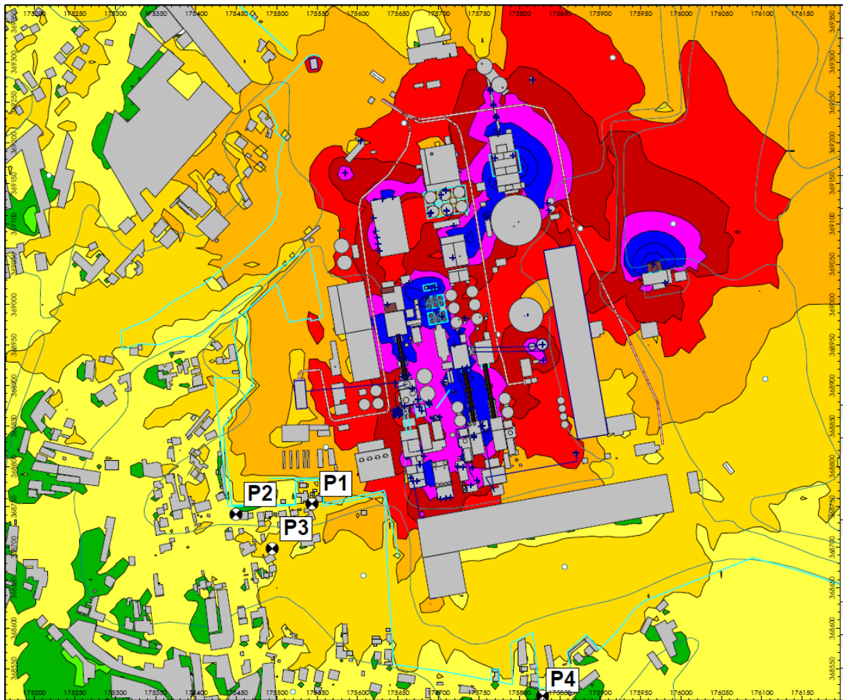
Figura 8-2 – Mapa de Ruído Particular do CPS da Cimpor para a Situação Futura – Cenário 1 (todas as fontes), a 4 m de altura – Ln.
