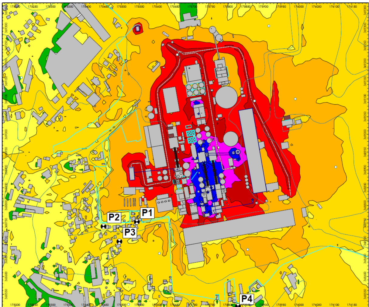
Figura 8-3 – Mapa de Ruído Particular do CPS da Cimpor para a Situação Futura – Cenário 2 (só com as fontes futuras), a 4 m de altura – Lden.
