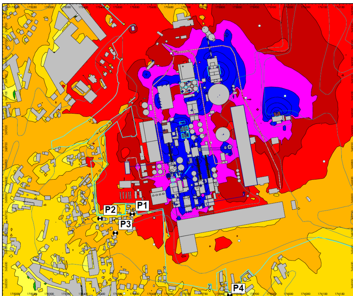
Figura 8-1 – Mapa de Ruído Particular do CPS da Cimpor para a Situação Futura – Cenário 1 (todas as fontes), a 4 m de altura – L_{den} .
