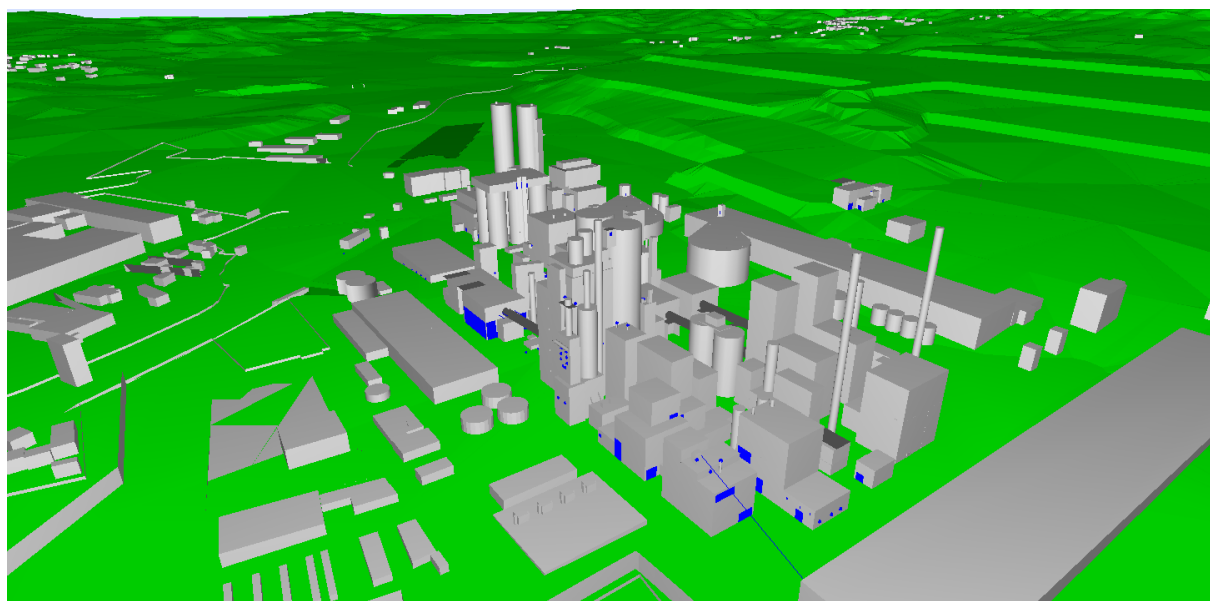
Figura 4-5 – Visualização 3D do modelo acústico criado versus vista 3D do Google Earth.
