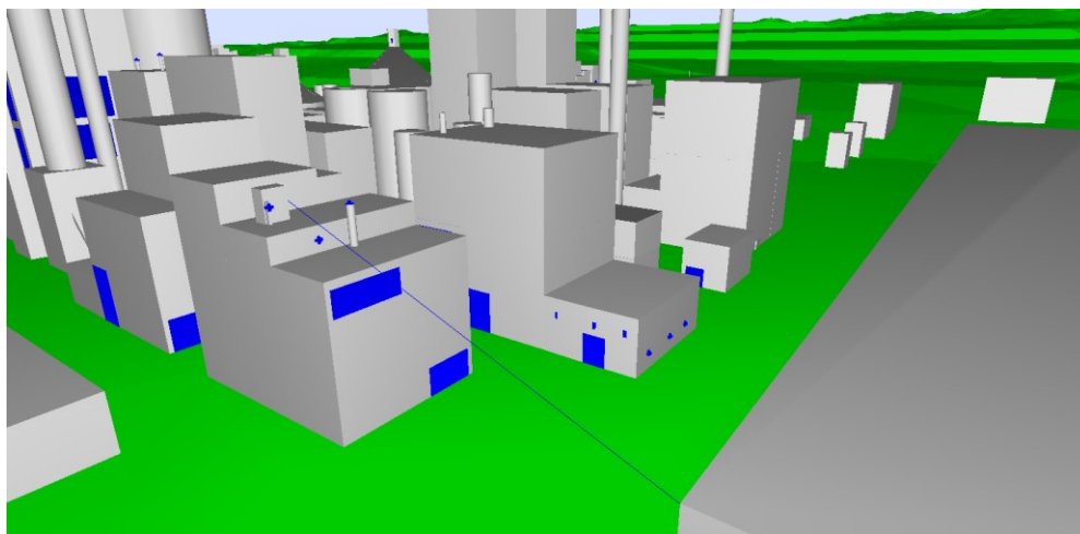
Figura 4-7 – Exemplo de fontes em área verticais (ex.: aberturas em edifícios), fontes pontuais (ex.: saída de chaminés, ventiladores) e fonte linear (tela transportadora).
