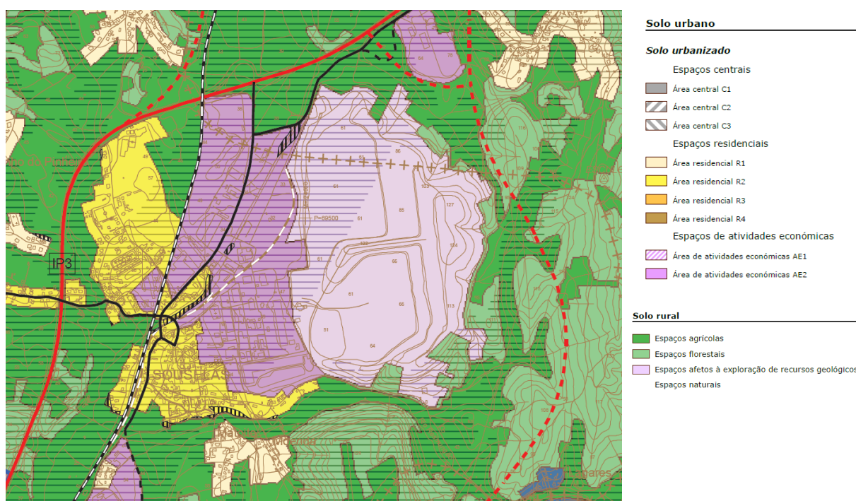
Figura 3-1 – Extrato da Planta de Ordenamento de Classificação e Qualificação do Solo.
