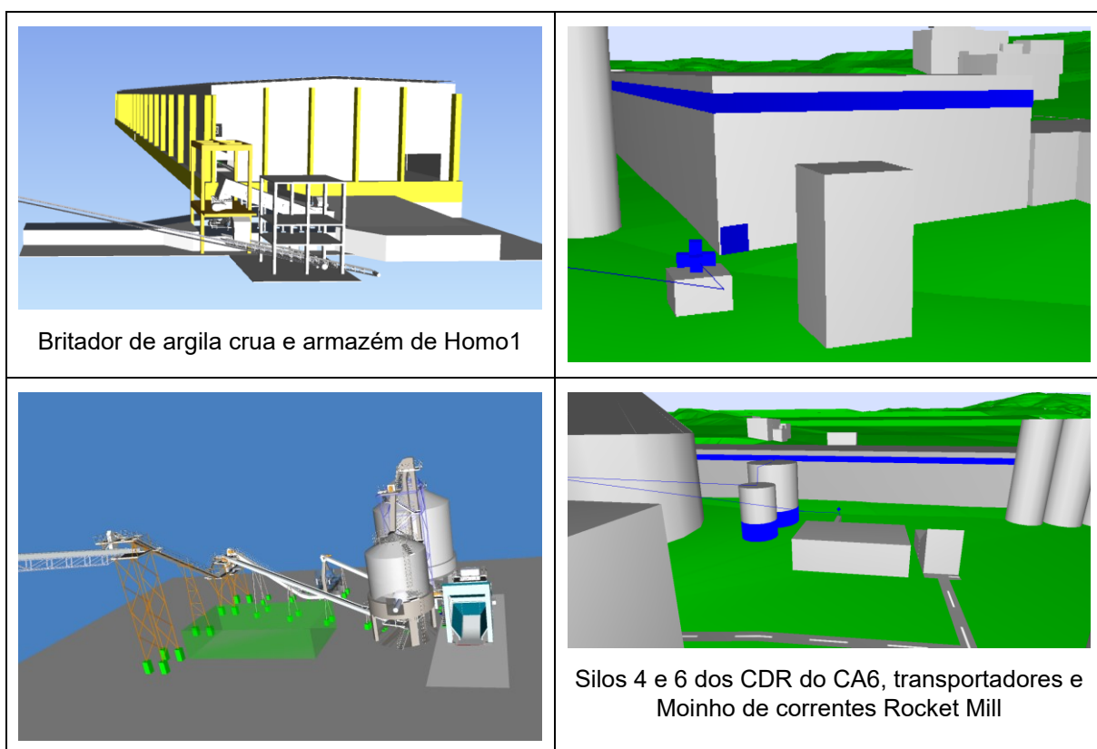
Figura 7-2 – Visualização 3D do modelo acústico criado para a situação futura (só representadas as fontes futuras).
