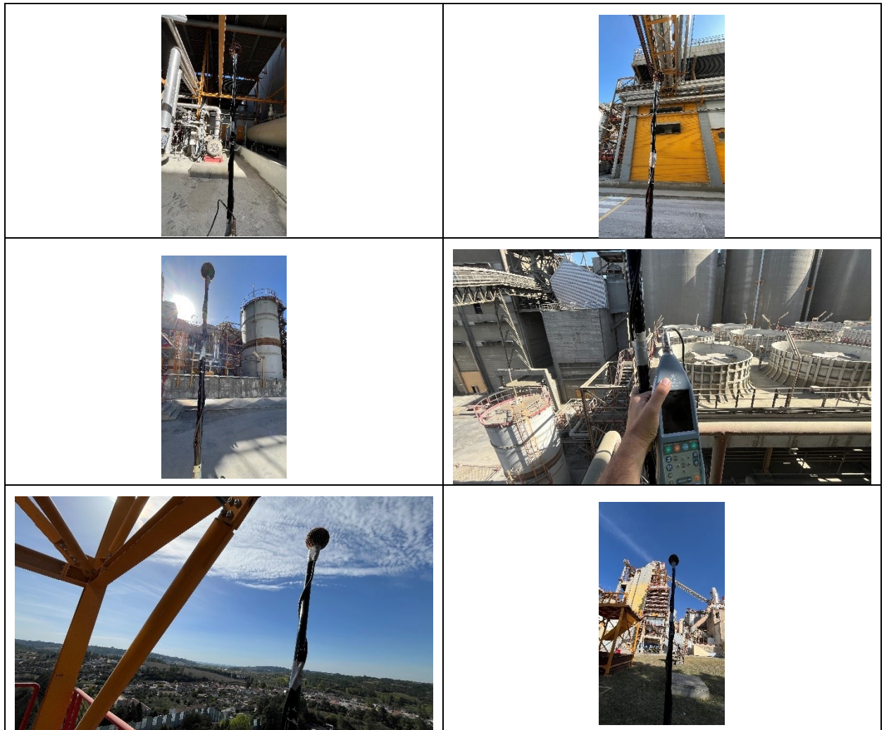
Figura 4-3 – Exemplos de medições de ruído para validação de fontes
