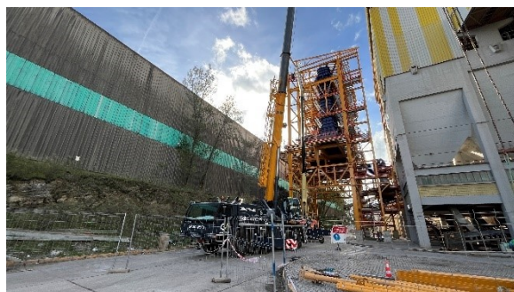
Tremonhas de argila crua, em construção, ao lado das tremonhas 1 e 2 existentes
