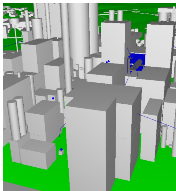
Tremonhas de argila crua, vendo-se os transportadores britador-tremonhas e tremonhas-secador; ao fundo o secador torre de ciclones e forno 2
