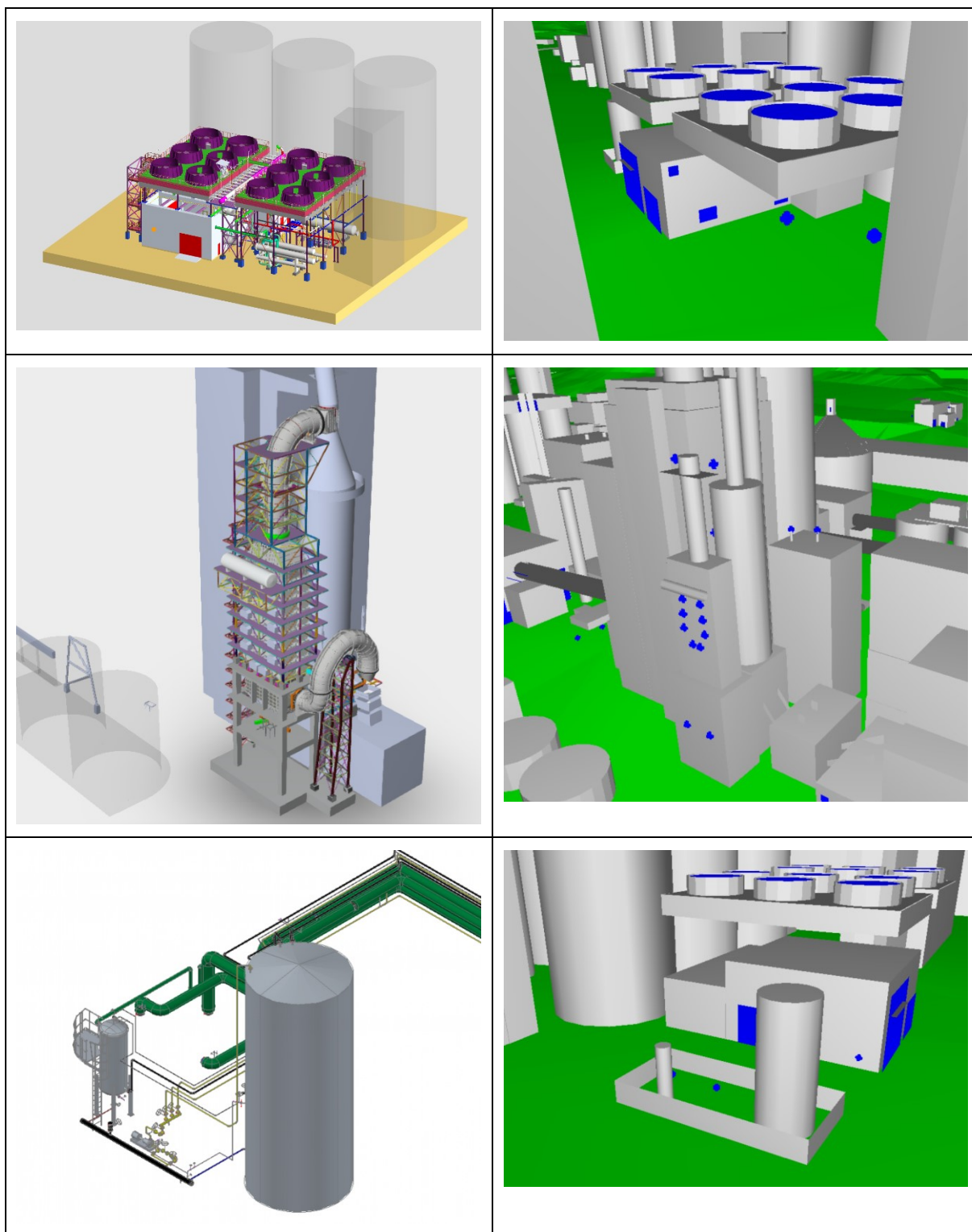
Figura 4-6 – Visualização de alguns dos modelos 3D de elementos do sistema WHR fornecidos pelo cliente e vistas correspondentes no modelo acústico desenvolvido: sala da turbina e condensadores de ar; pré-aquecedor; pít com bombas de fluido térmico, depósito e vaso de expansão.
