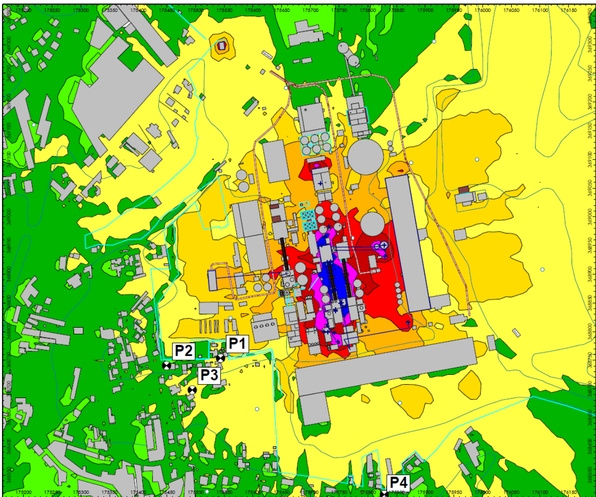
Figura 8-4 – Mapa de Ruído Particular do CPS da Cimpor para a Situação Futura – Cenário 2 (só com as fontes futuras), a 4 m de altura – Ln.
