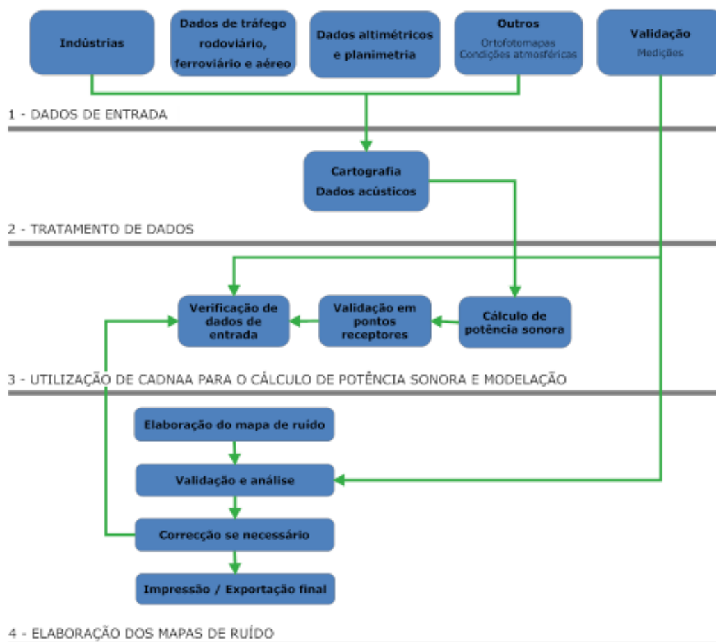
Figura 4-1 – Diagrama da metodologia geral utilizada pela dBwave.i para a elaboração de mapas de ruído
