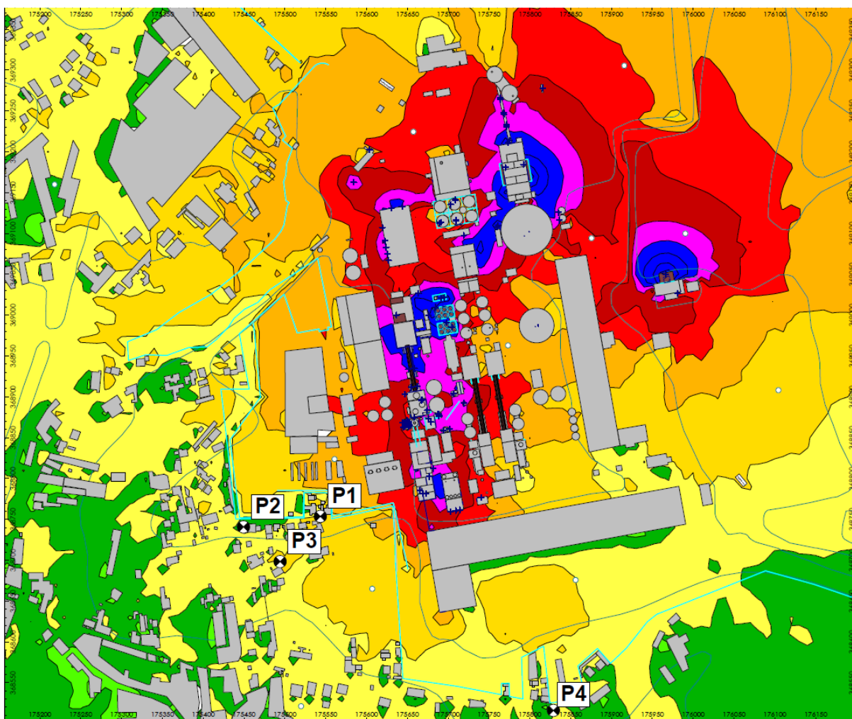
Figura 5-3 – Mapa de Ruído Particular do CPS da Cimpor a Outubro 2025, a 4 m de altura – Ln.
