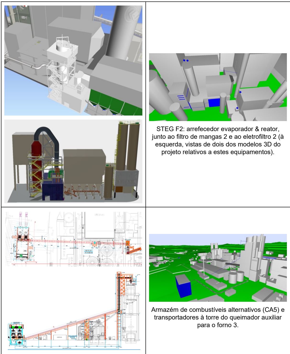
Figura 7-3 – Visualização de alguns dos desenhos e modelos 3D dos projetos no âmbito do EIA fornecidos pelo cliente e vistas correspondentes no modelo acústico desenvolvido.
