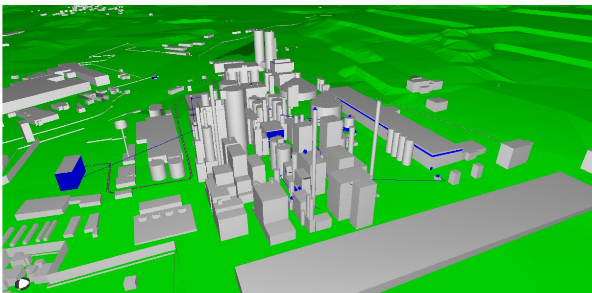
Figura 7-2 – Visualização 3D do modelo acústico criado para a situação futura (só representadas as fontes futuras).
