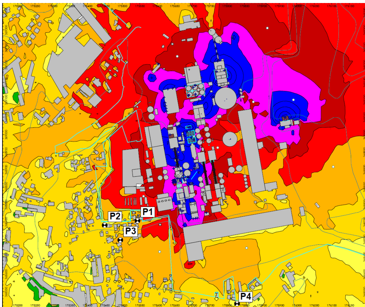
Figura 5-2 – Mapa de Ruído Particular do CPS da Cimpor a Outubro 2025, a 4 m de altura – Lden.
