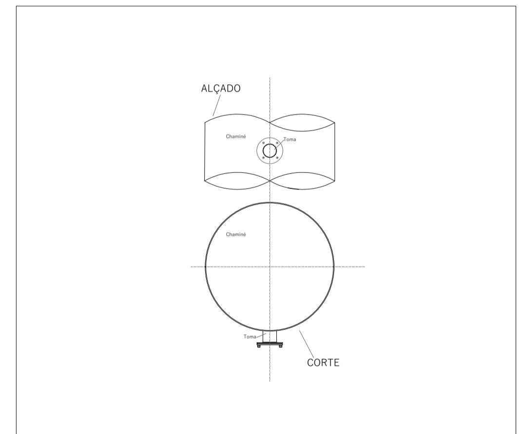
FORMENOR CHAMINÉ Escala 1/10
