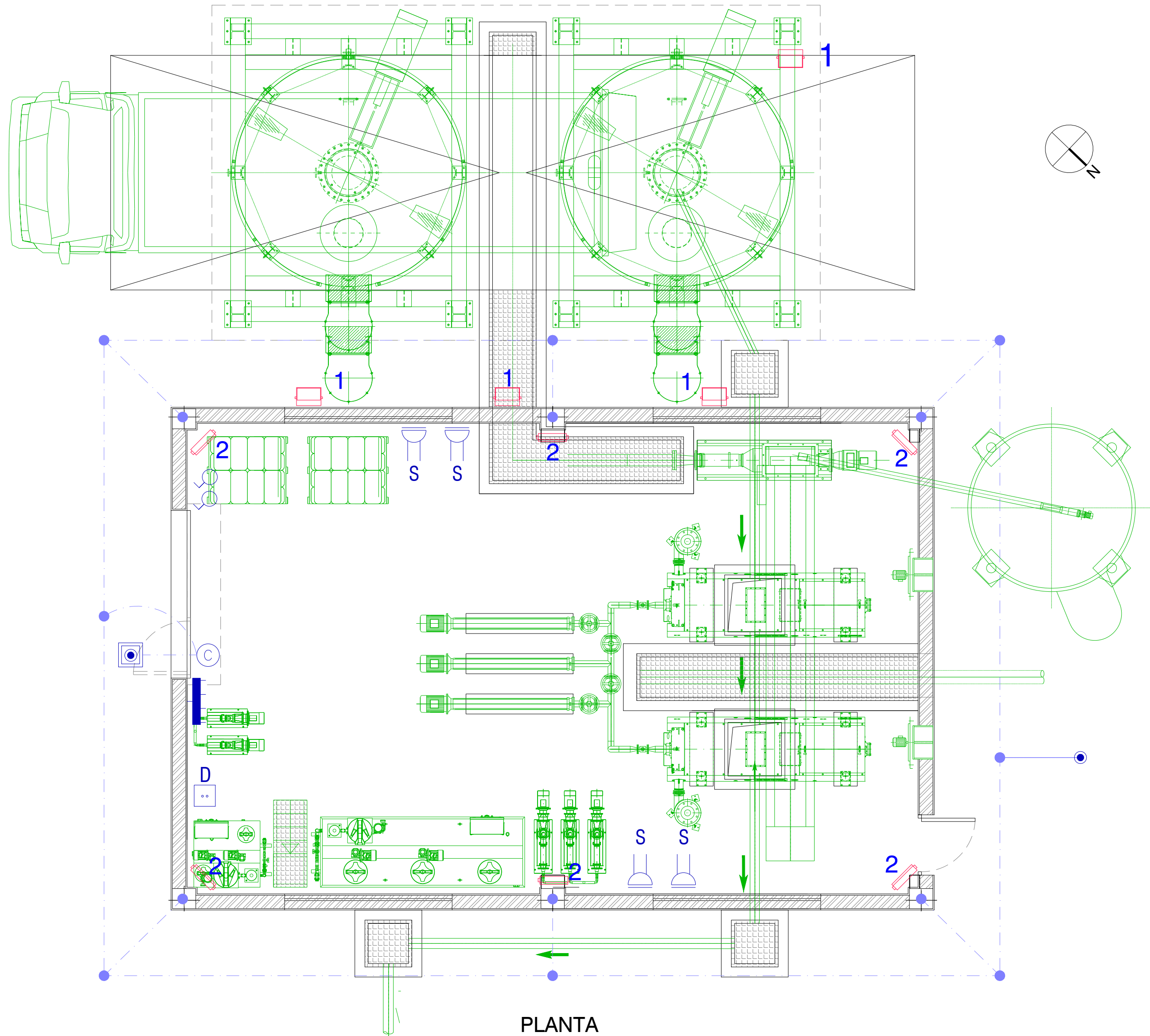
PLANTA Esc: 1:50 (A1) Esc: 1:100 (A3)
