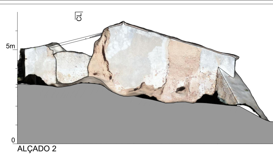
ALÇADO 2
