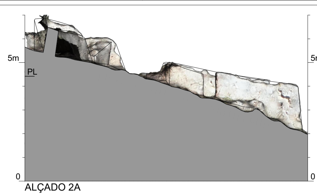
ALÇADO 2A
