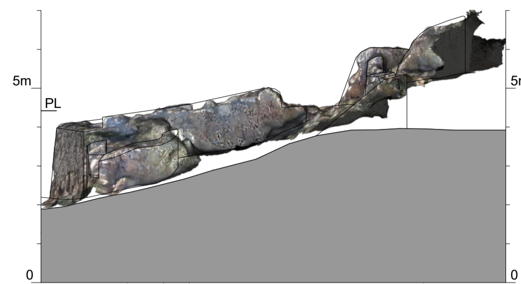
ALÇADO 3A
