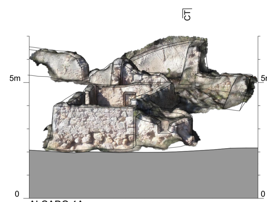
ALÇADO 1A
