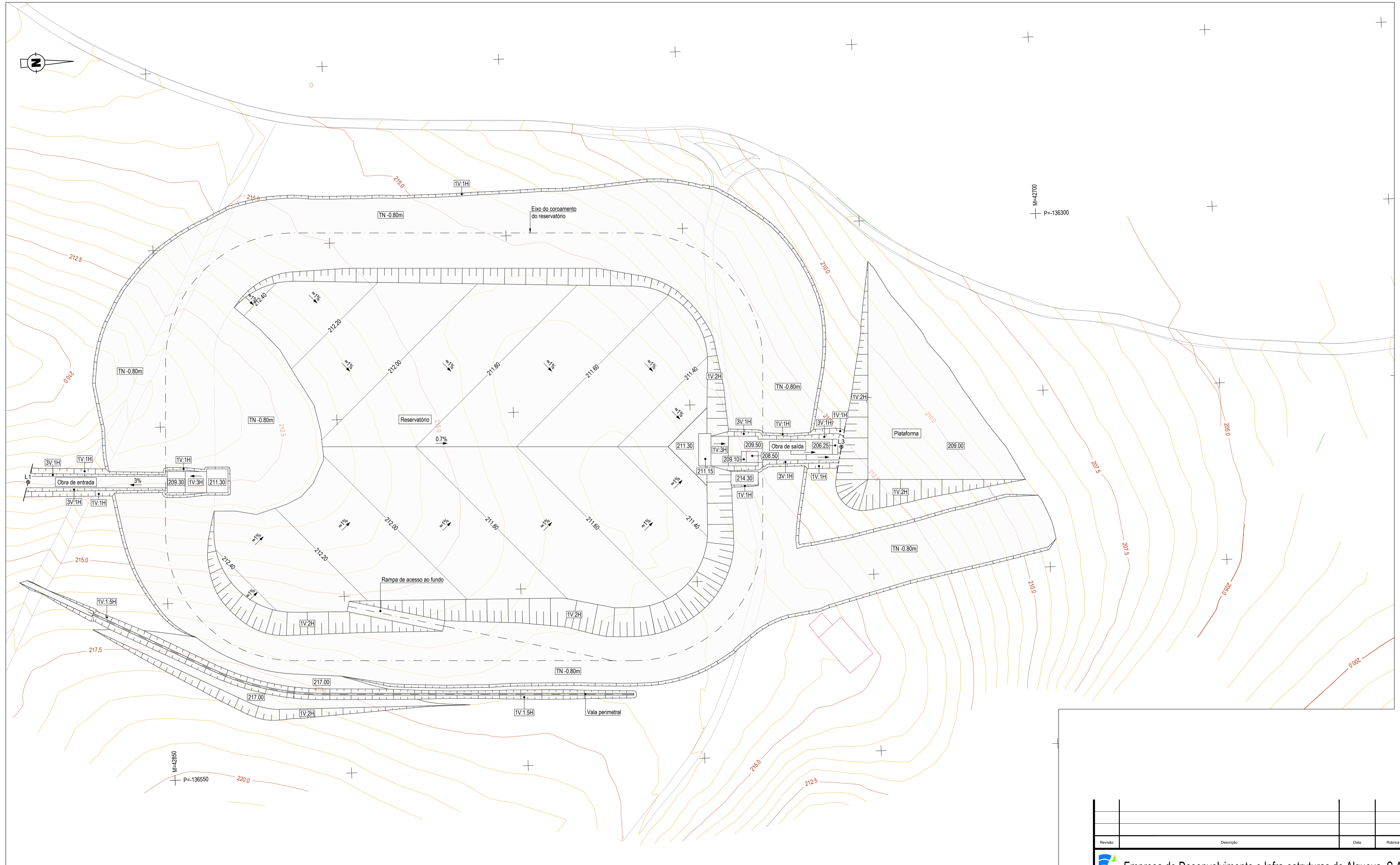
PLANTA Esc. 1:500
