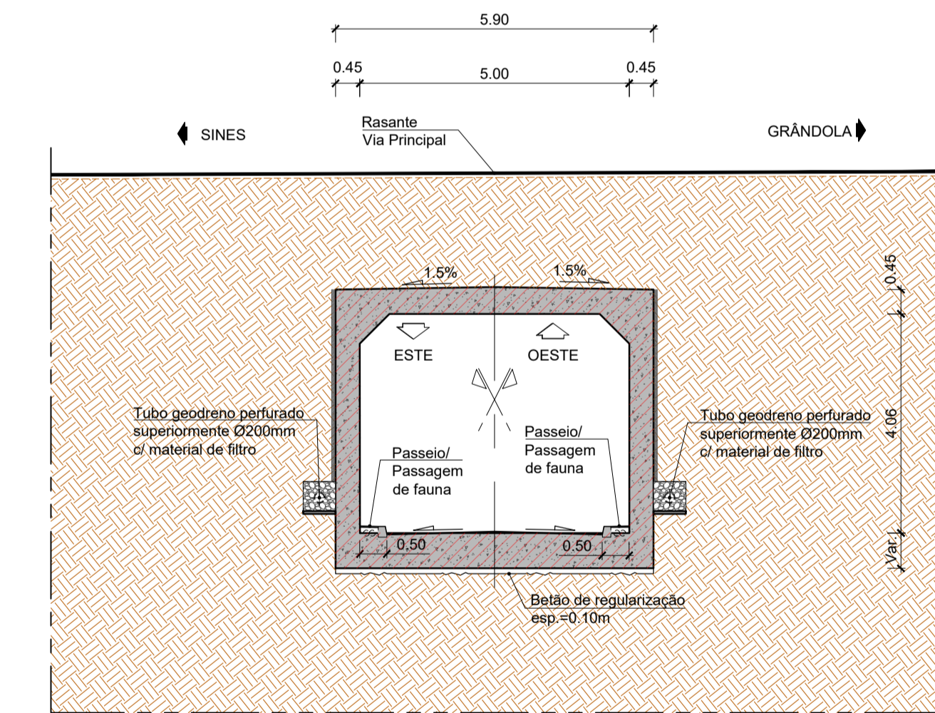
CORTE C-C ESC=1:100
