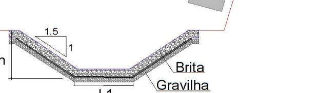
Corte esquemático da Rede de Drenagem dos Taludes
