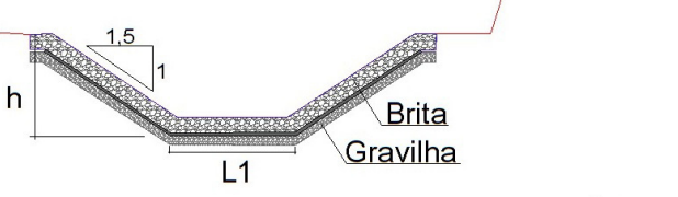
Corte esquemático da Rede de Drenagem dos Taludes
