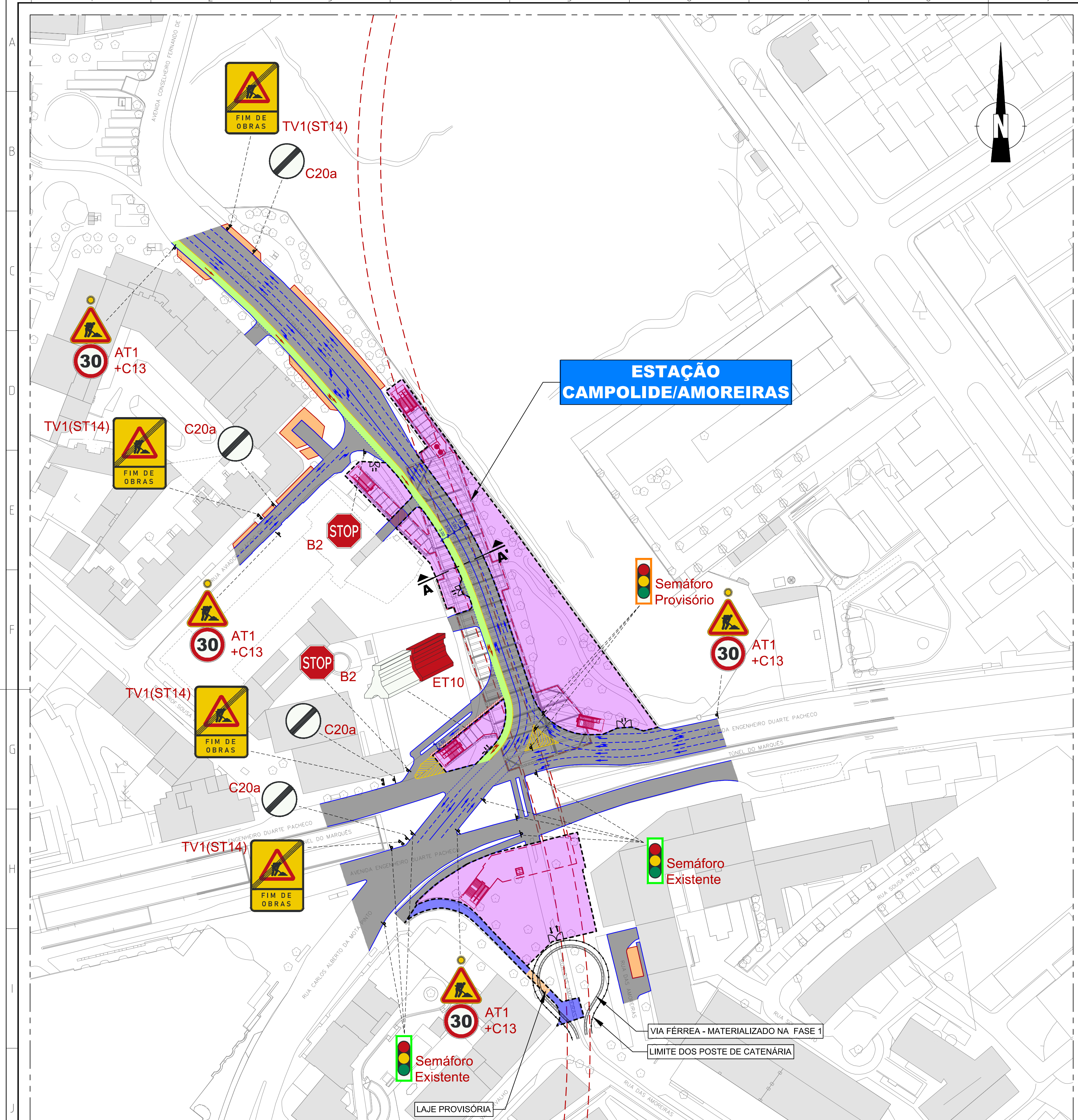
PAVIMENTO DEFINITIVO DE CIRCULAÇÃO VIÁRIA ESC. 1:10
