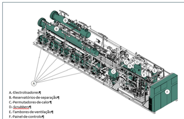
Figura 4 - Vista do módulo de processo da electrólise da água
