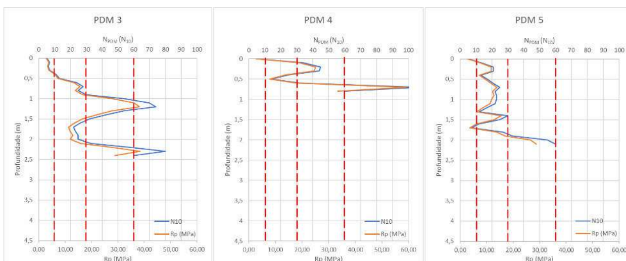
Figura 35 - Resultados obtidos no alinhamento PDM 3 – PDM 4 – PDM 5 ( N_{10} e R_p ). As linhas vermelhas representam os intervalos considerados na análise patente no Quadro 16
