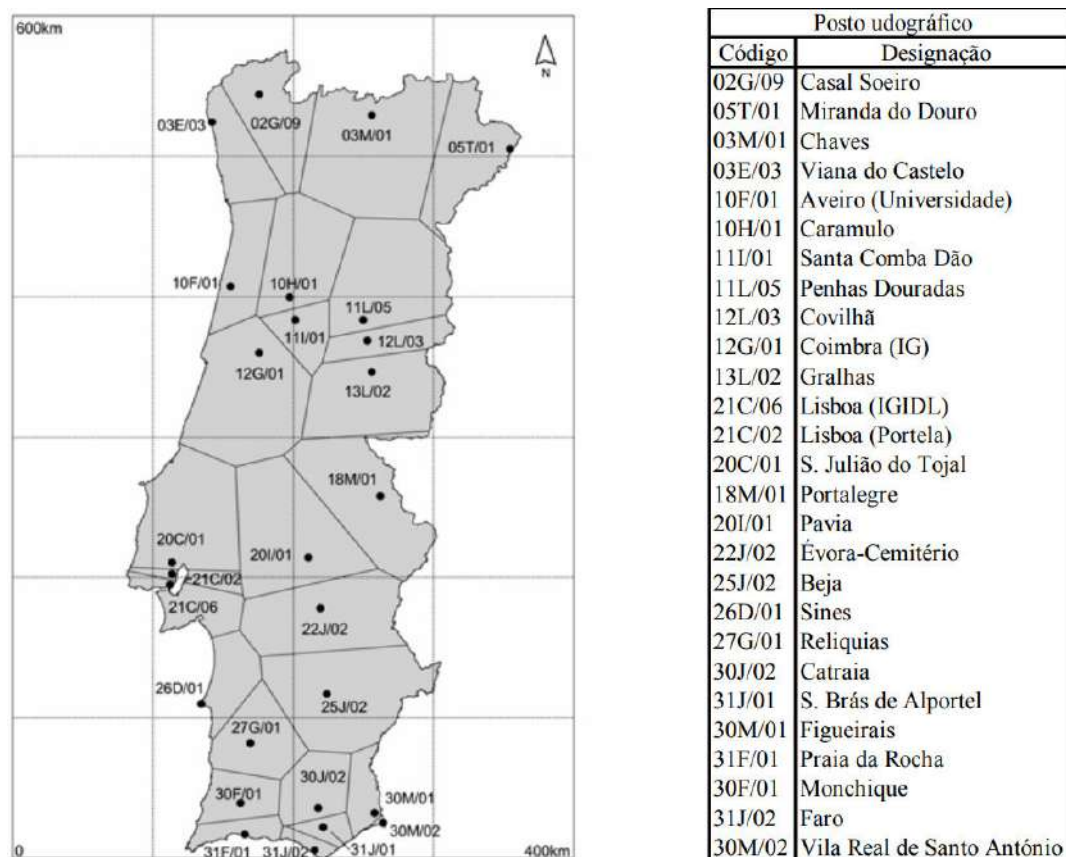
Figura 3.1 – Polígonos de Thiessen para os 27 postos udográficos utilizados no estudo de Brandão et al (2001)
