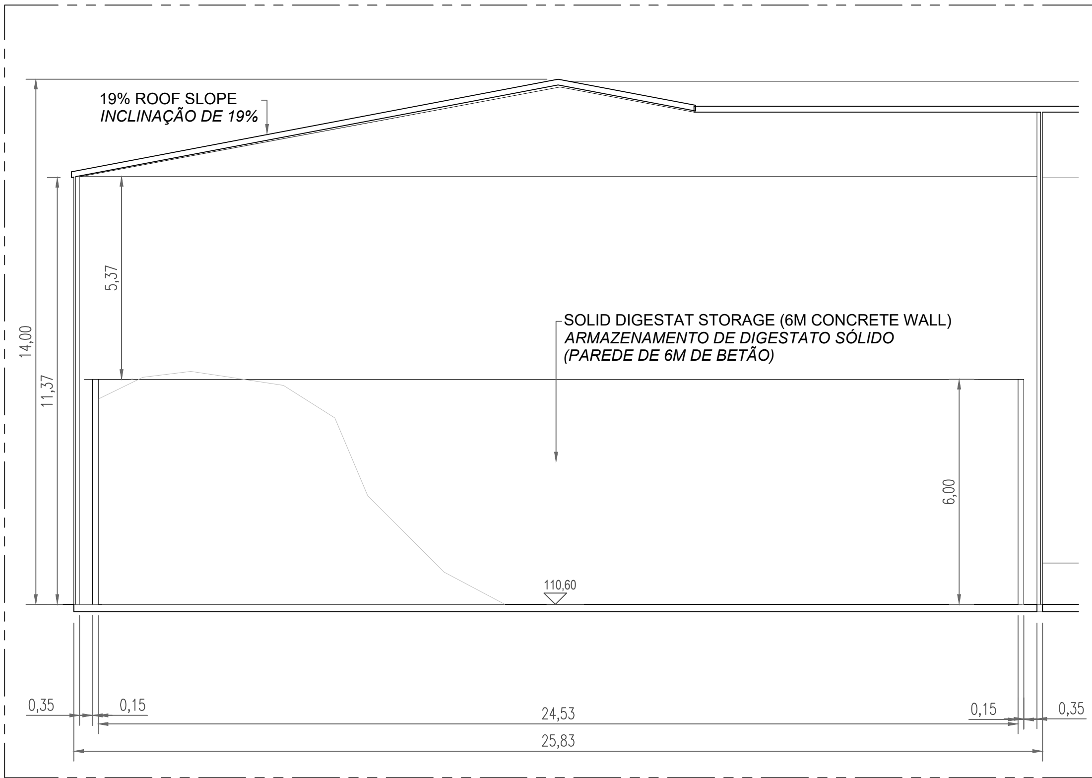
CORTE 05 ESCALA 1:100
