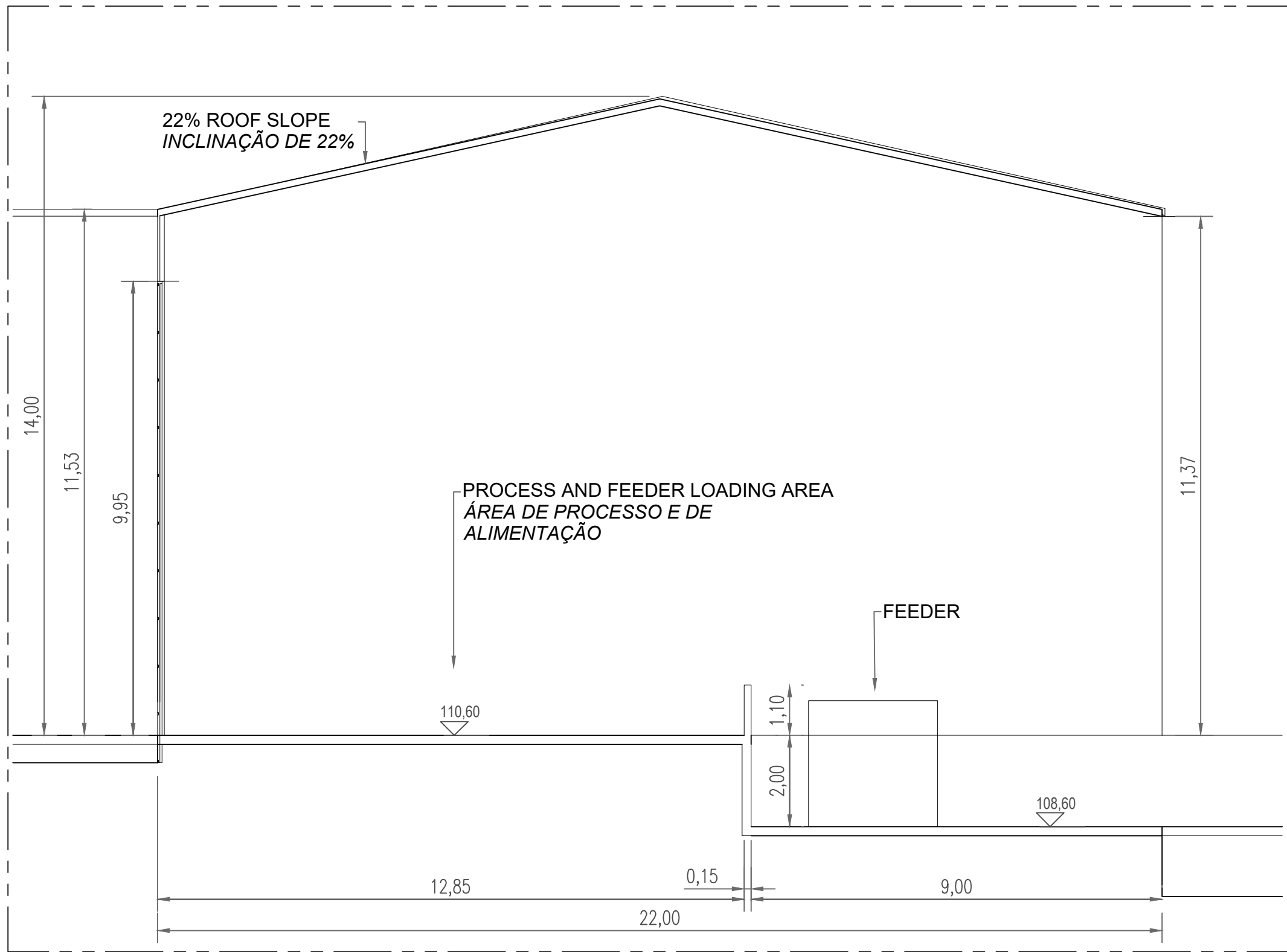
CORTE 04 ESCALA 1:100
