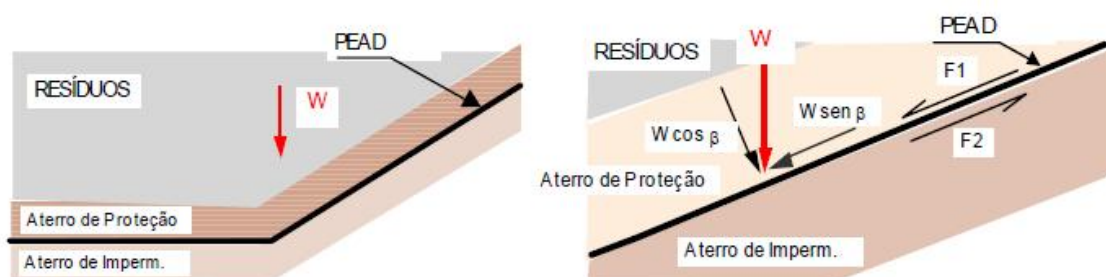
Figura 1 – Diagrama dos esforços de tração aplicados na geomembrana
