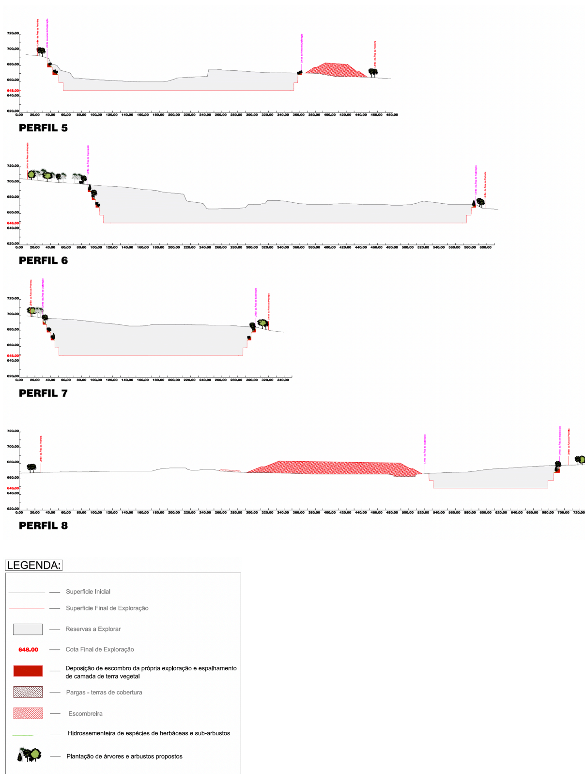
Figura 173: Perfis iniciais e finais de exploração da Pedreira n.º 5419 “Ervilhão”.
