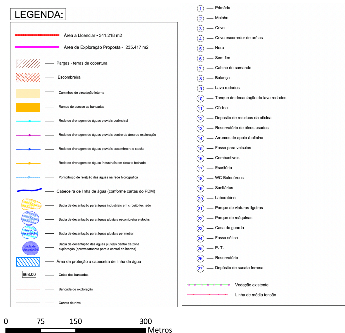
Figura 14: Rede de drenagem
