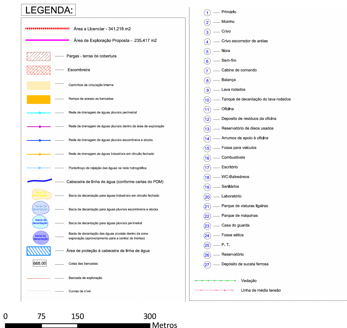
Figura 3: Plano de lavra – Situação final da exploração.
