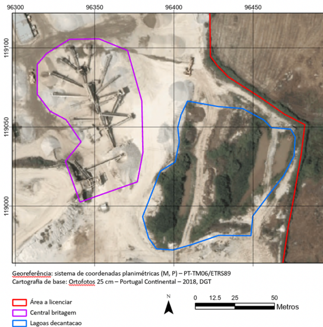
Figura 13: Fotografia aérea da lagoa de decantação e da central de britagem e de areias.
