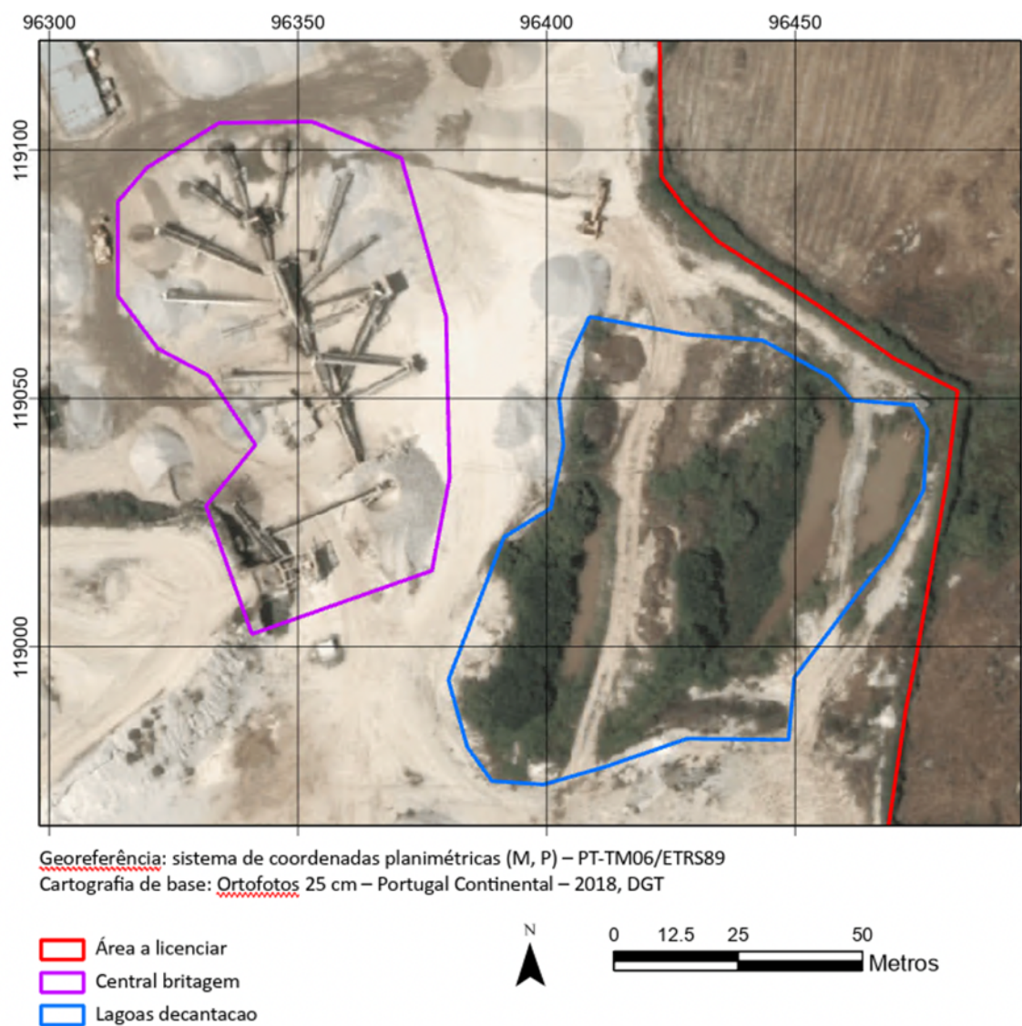
Figura 107: Fotografia aérea da lagoa de decantação e da central de britagem e de areias.
