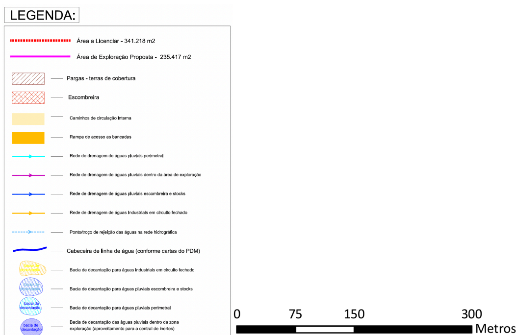
Figura 15: Situação final de exploração da Pedreira n.º 5419 “Ervilhão”.
