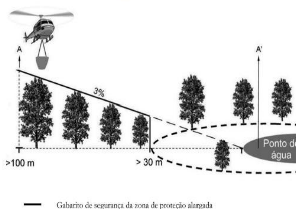
Figura 3: Gabarito de segurança a respeitar na zona de proteção alargada do cone de voo de aproximação (perfil longitudinal do corte A-A' da figura 2). A ZPA representada deve ser também aplicada ao cone de voo de saída e à escapatória de emergência.
