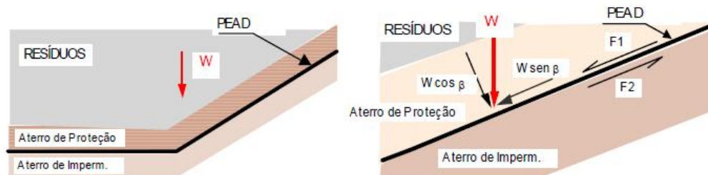
Figura 4 – Diagrama dos esforços de tração aplicados na geomembrana
