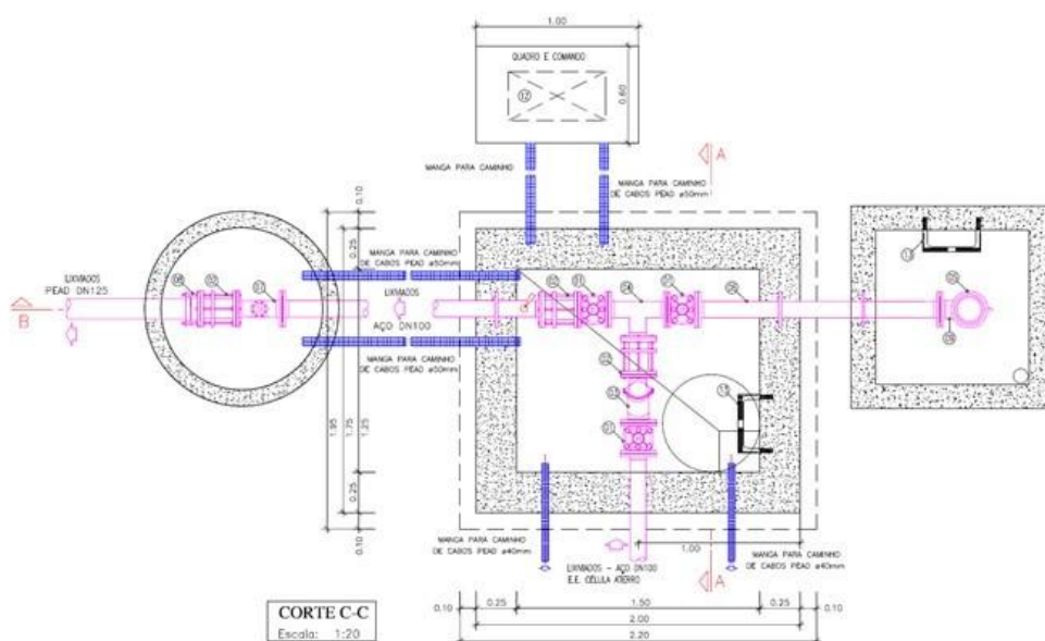
Figura 6 - Caixa de medição de caudal, caixa das válvulas e caixa de descarga de fundo
