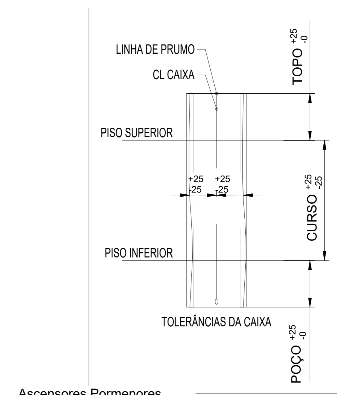
Ascensores Pormenores
