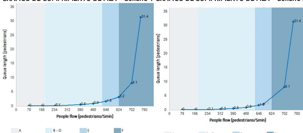
GRÁFICO DE COMPRIMENTO DE FILA – Cenário 1 GRÁFICO DE COMPRIMENTO DE FILA – Cenário 2
