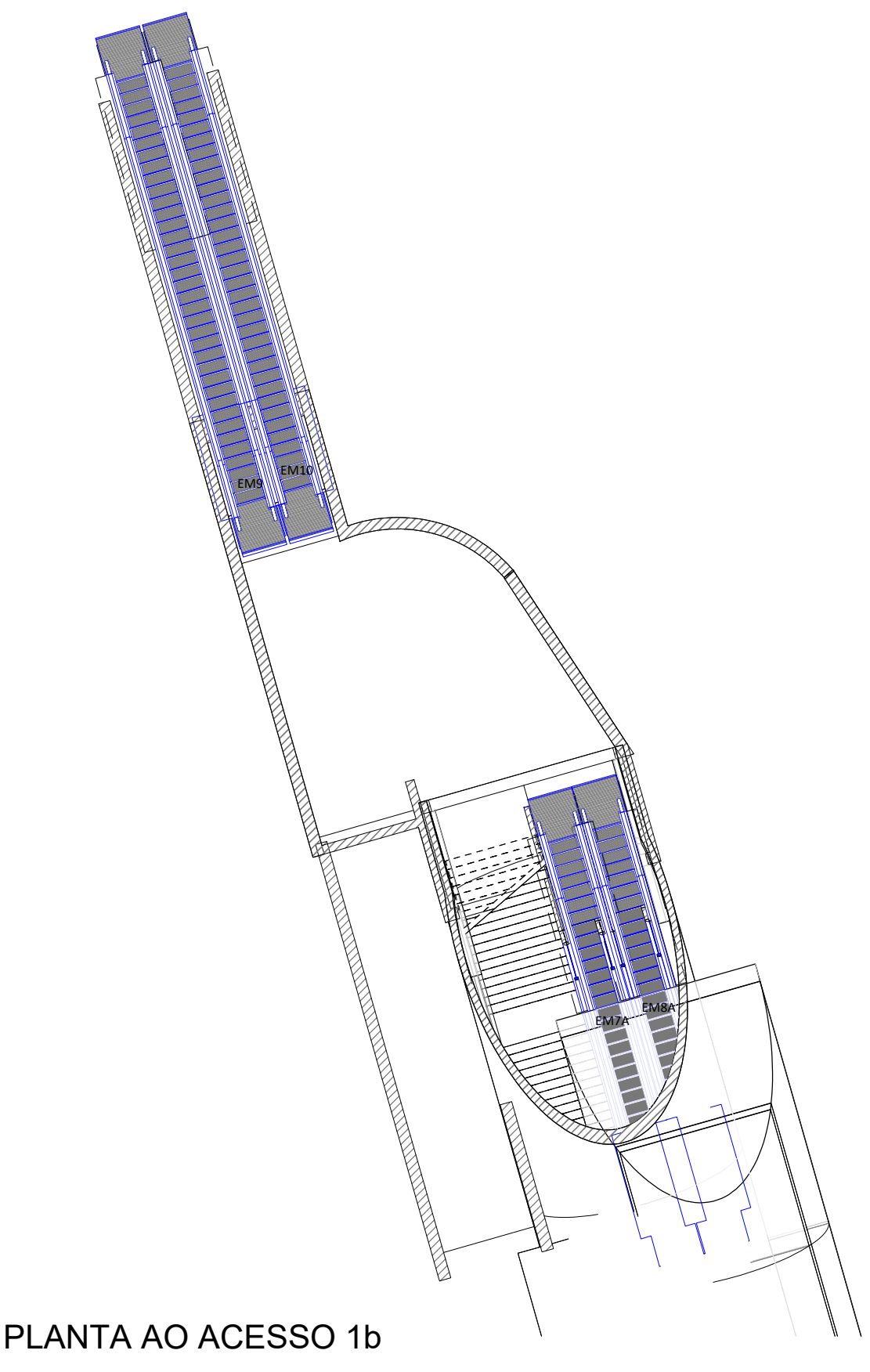
PLANTA AO ACESSO 1b
