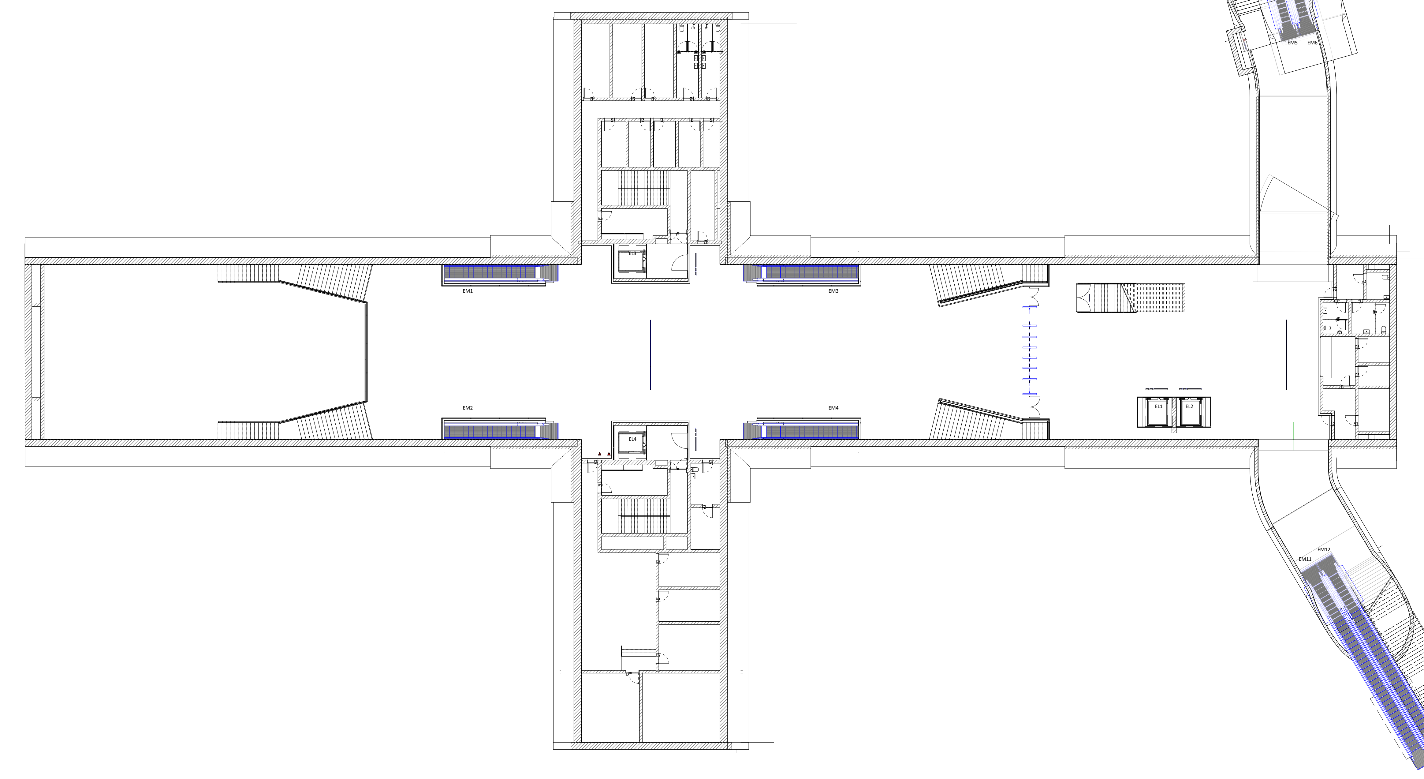
PLANTA AO NÍVEL ÁTRIO
