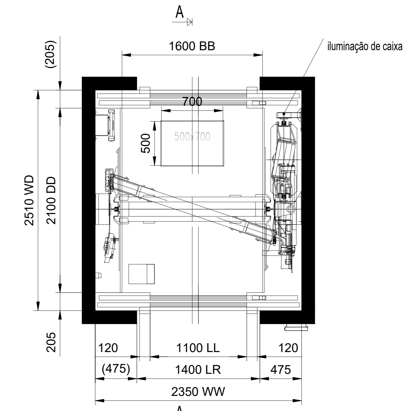
CABINA E PLANO DA CAIXA
