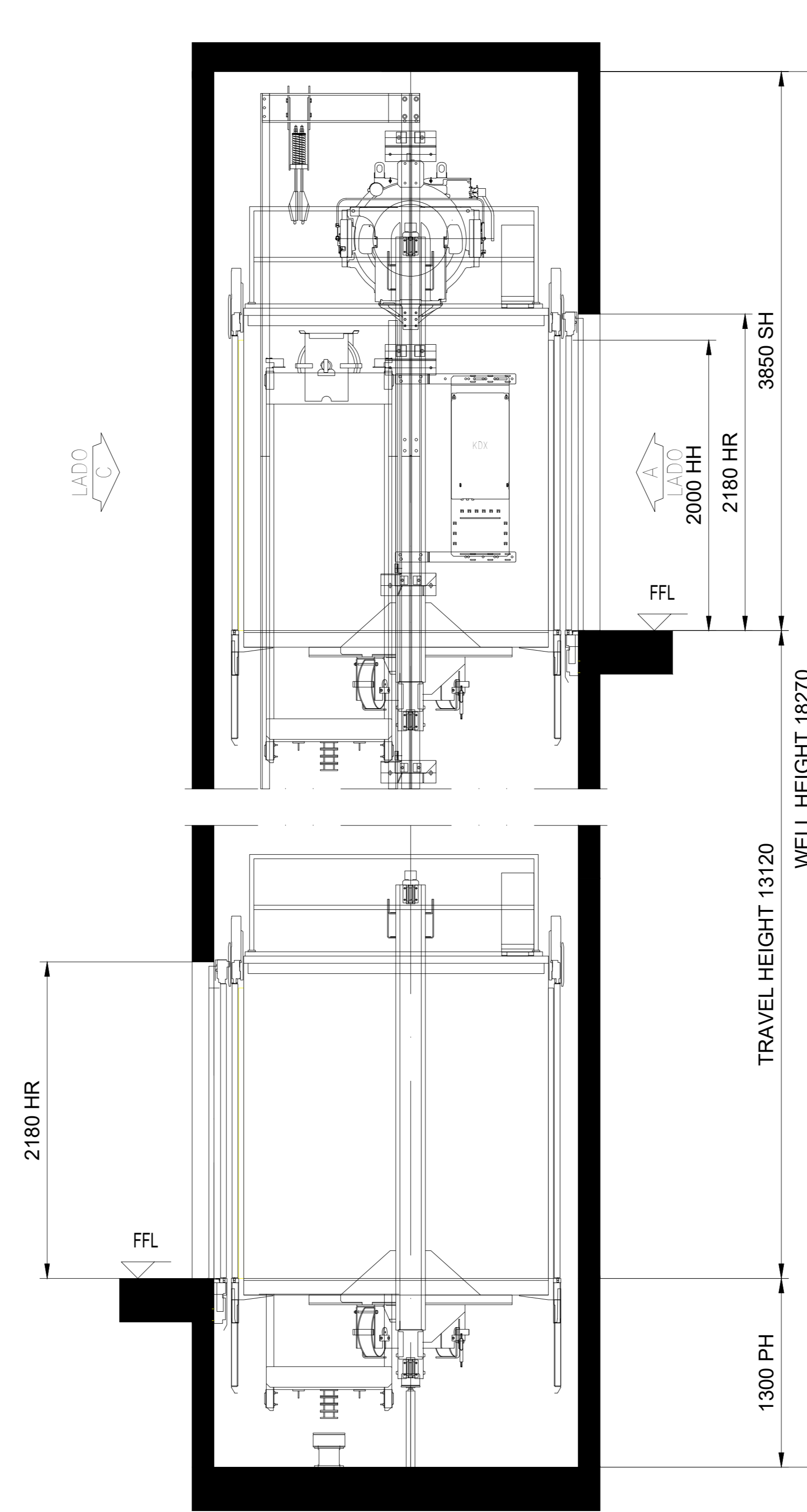
SECÇÃO A-A
