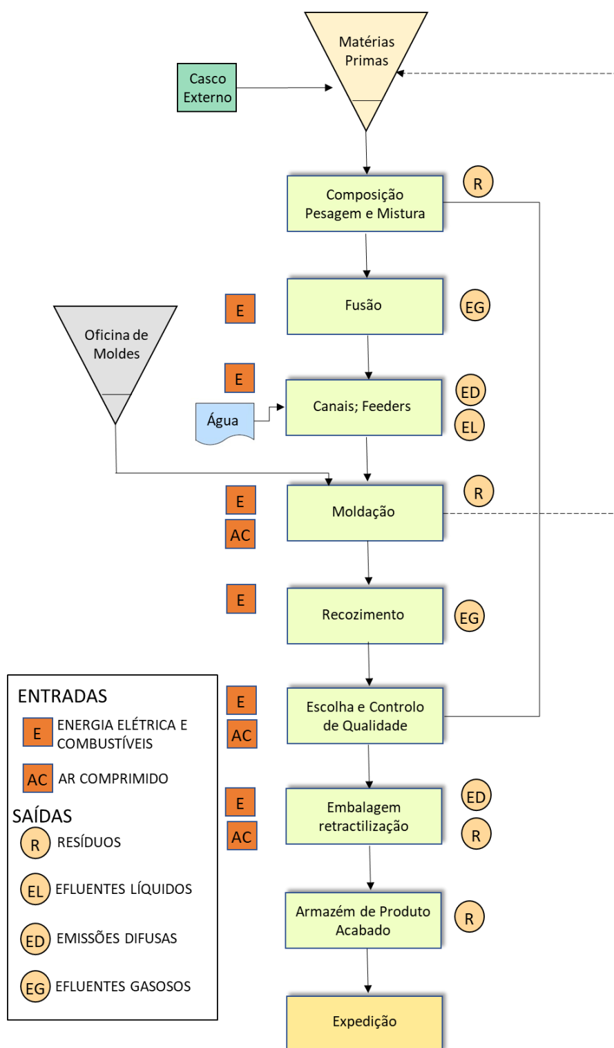
Fluxograma do processo produtivo de fabrico de vidro de embalagem
