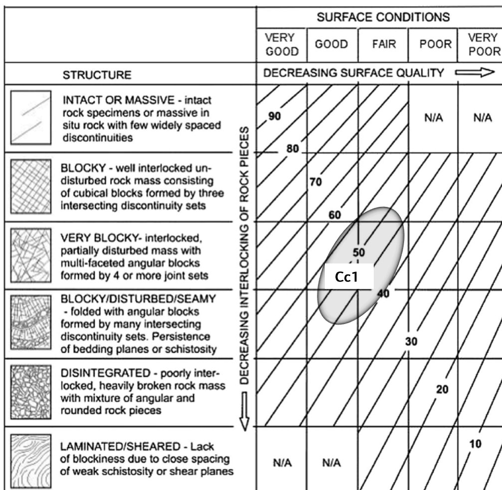
Figura 26 - Unidade Geotécnica Cc1c - gama de valores representativos de IGS
