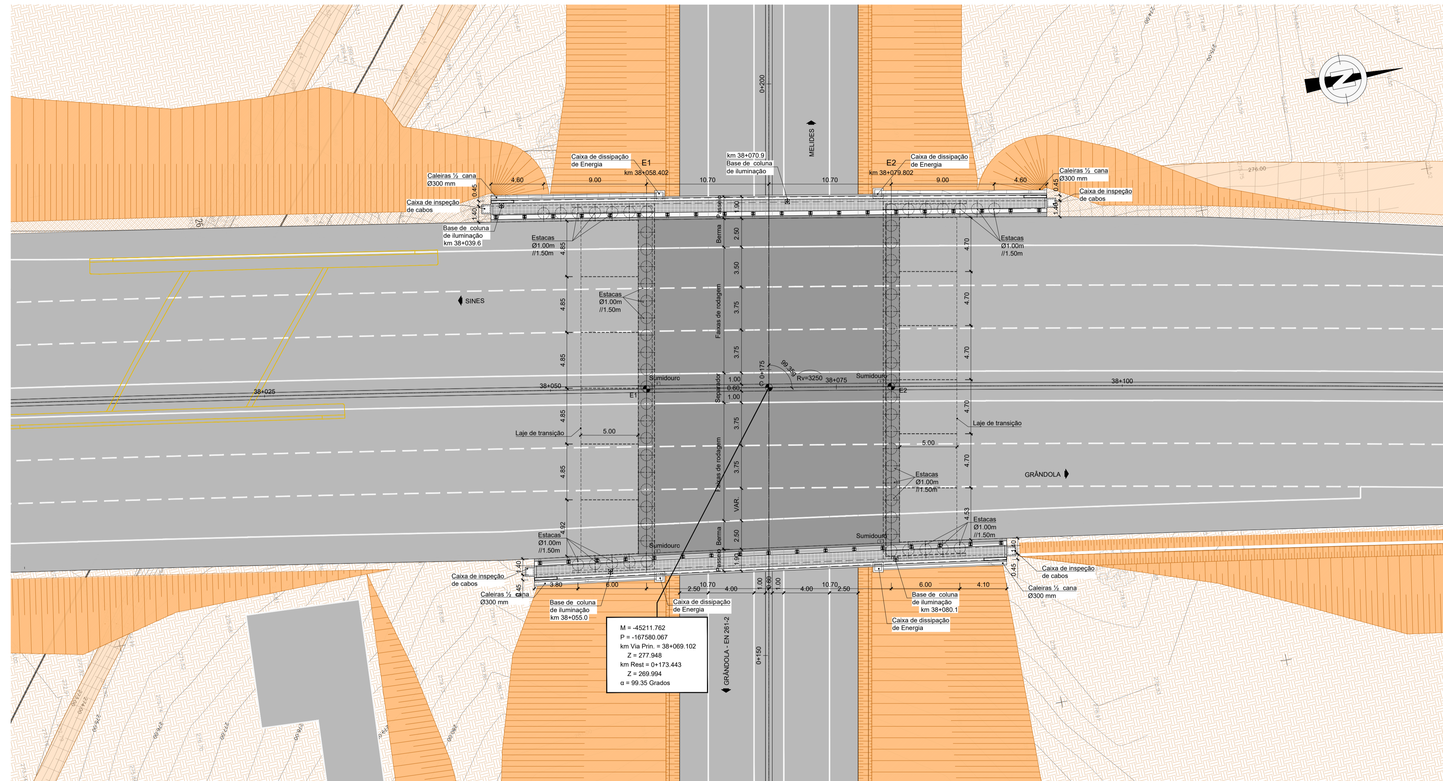
PLANTA ESC=1:200
