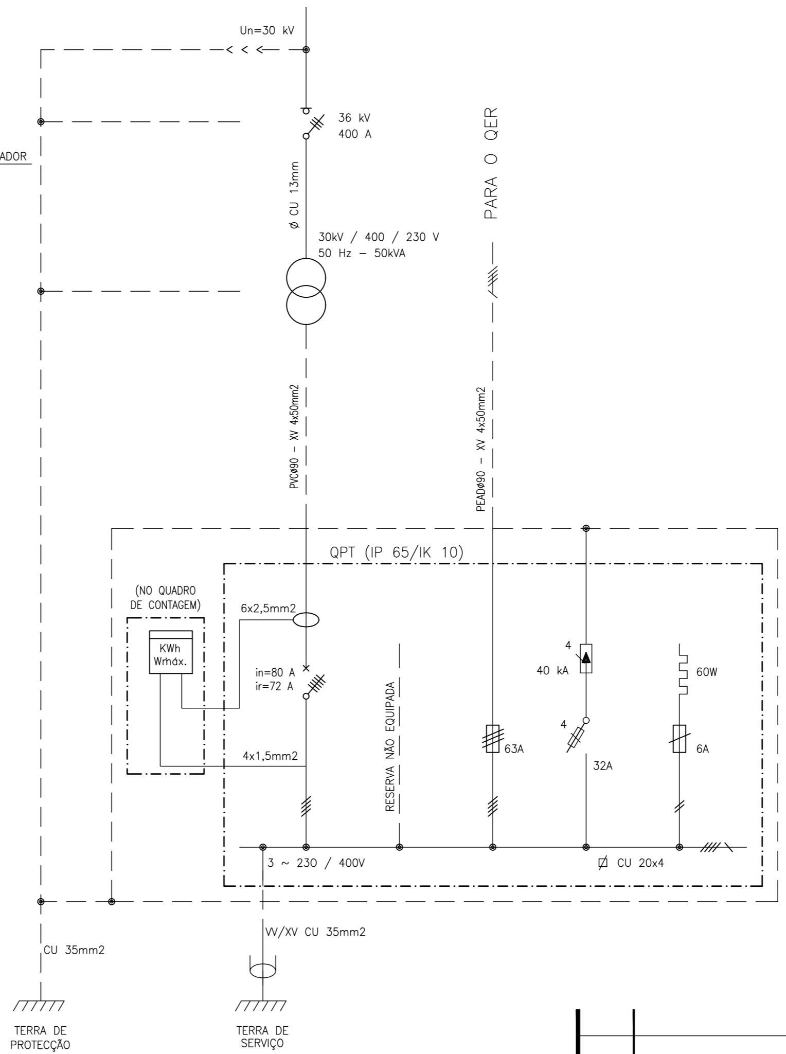
P.T. AÉRIO RURAL - AS 50 kVA - 30 kV ± 5 % - 400 / 230 V
