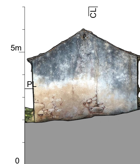
ALÇADO 4
