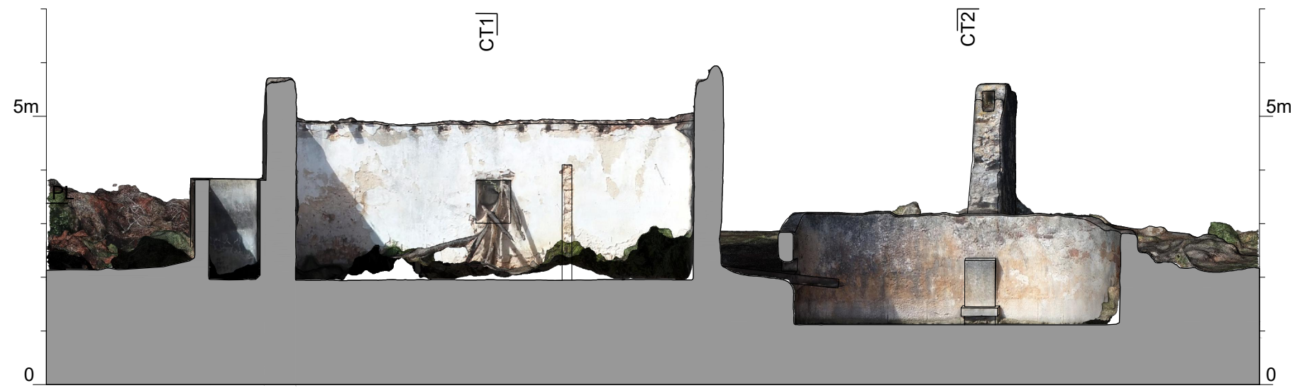
CORTE LONGITUDINAL
