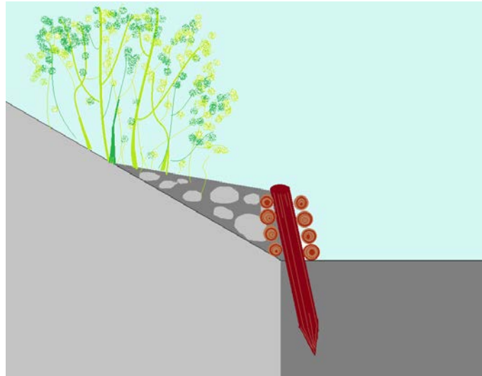
Figura 6.2 – Técnica de Bioengenharia: Entrançado.
