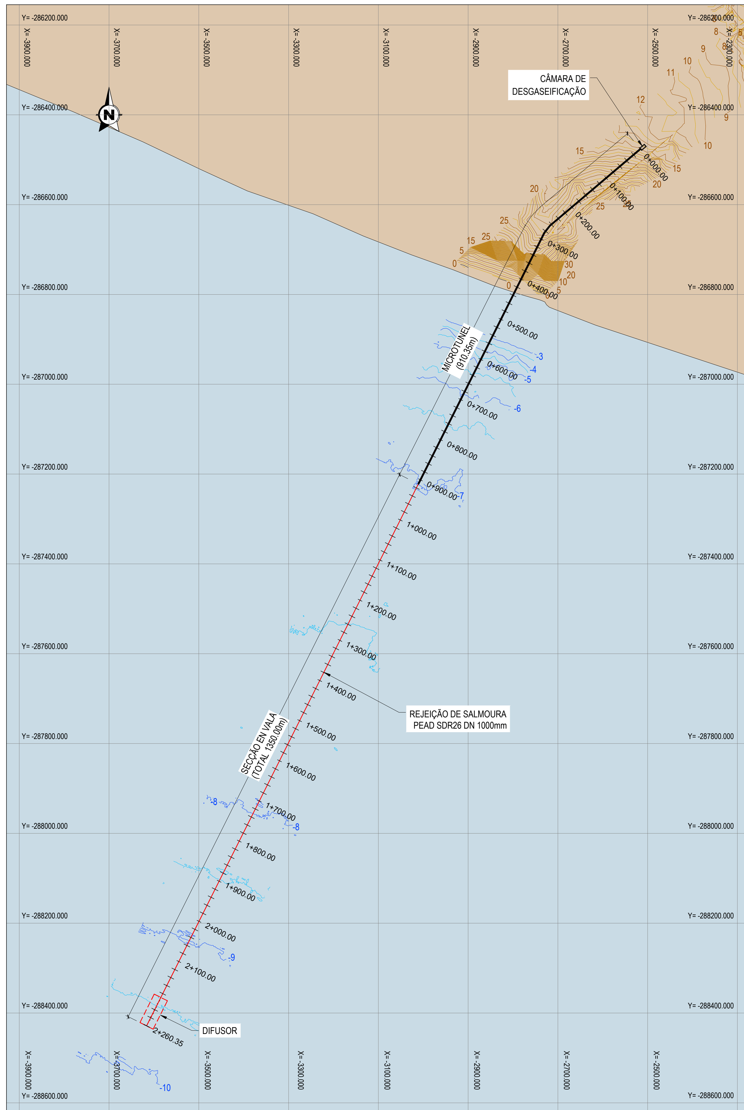
PLANTA GERAL REJEIÇÃO DE SALMOURA ESCALA 1:5.000
