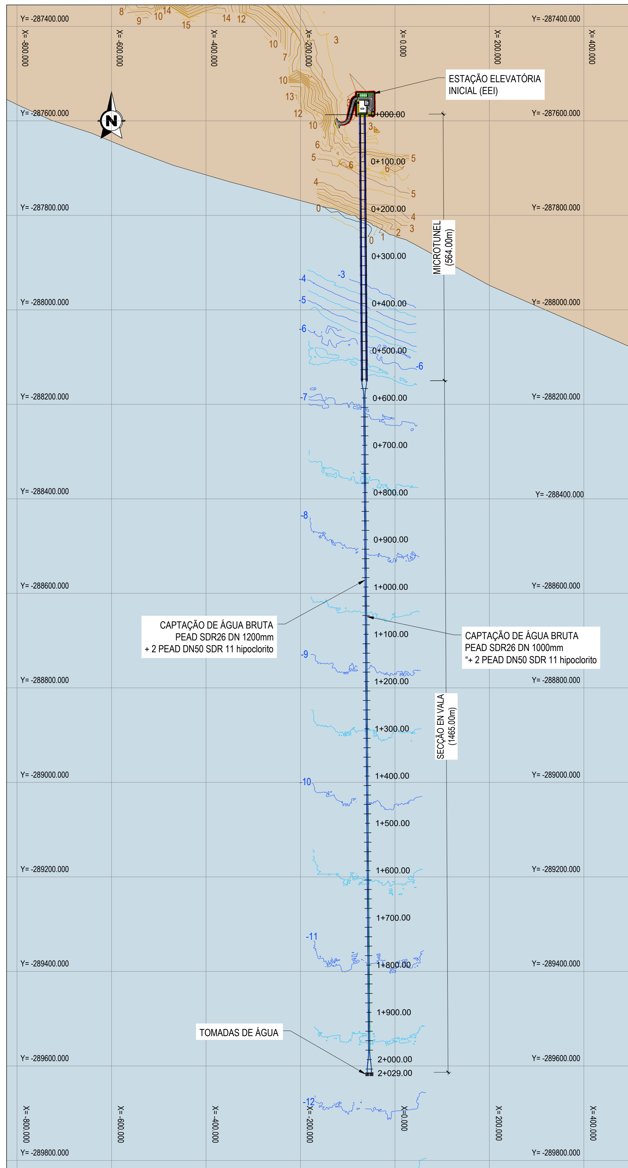
PLANTA GERAL CAPTAÇÃO DE ÁGUA BRUTA ESCALA 1:5.000
