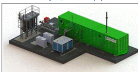
Figura III.20 – Vista do arranjo típico dos equipamentos de upgrading
