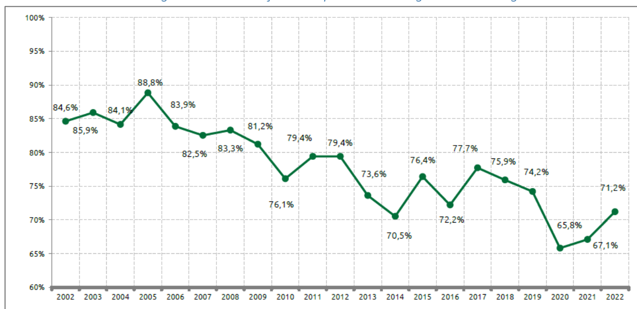
Figura V.14 – Evolução da dependência energética em Portugal
