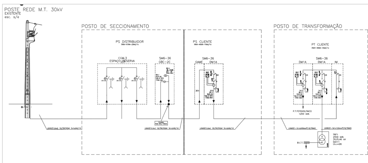
Figura III.3 – Esquema da ligação da rede pública ao posto de seccionamento da instalação
