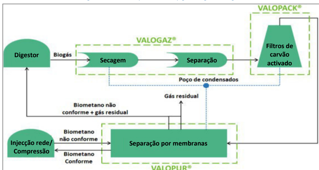
Figura III.19 – Esquema do upgrading do biogás
