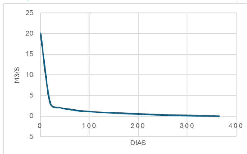
Figura IV.34 – Curva de duração média anual do caudal médio diário – ribeira Grande (estação 19M/01H)
