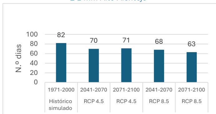
Figura IV.20 – N.º de dias com precipitação \geq 1 \text{ mm} Alto Alentejo
