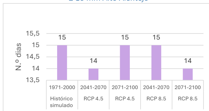
Figura IV.21 – N.º de dias com precipitação \geq 10 \text{ mm} Alto Alentejo
