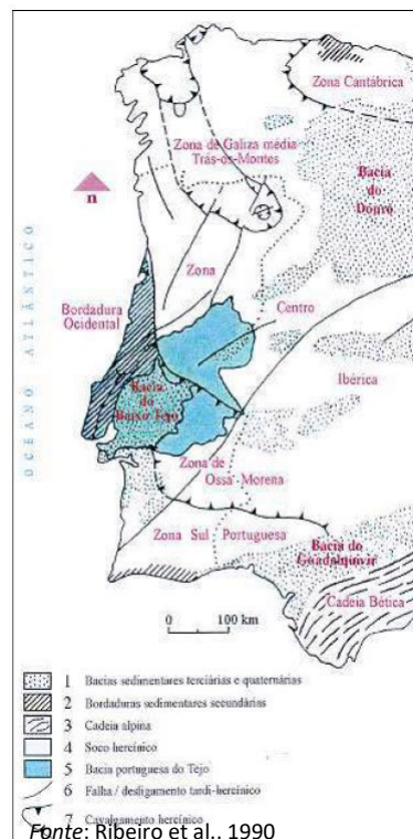
Figura IV.23 – Zonamento tectono-estratigráfico do Maciço Hespérico
