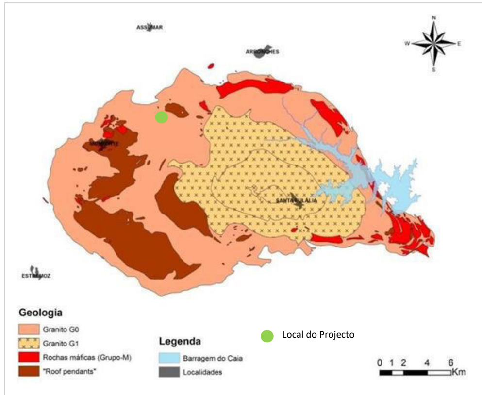
Figura IV.25 – Complexo Plutónico de Santa Eulália
