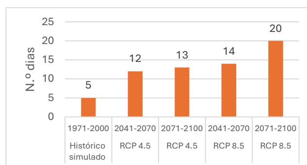
Figura IV.17 – Duração média da onda de calor Alto Alentejo
