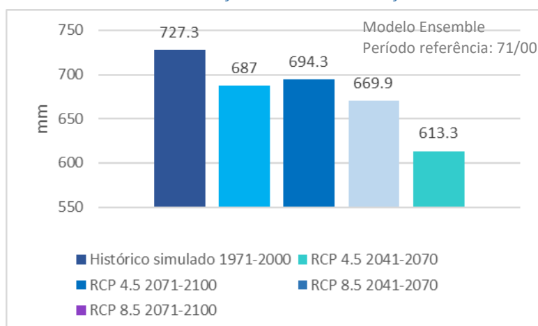
Figura IV.14 – Precipitação média anual no clima actual e nos cenários futuros – Alto Alentejo
