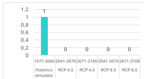
Figura IV.19 – Duração da onda de frio Alto Alentejo
