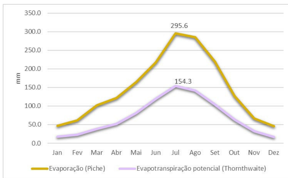
Figura IV.5 – Normais climatológicas dos valores de evaporação registados na Estação Meteorológica de Elvas, no período 1971-2000. Evapotranspiração calculada pelo método de Thornthwaite
