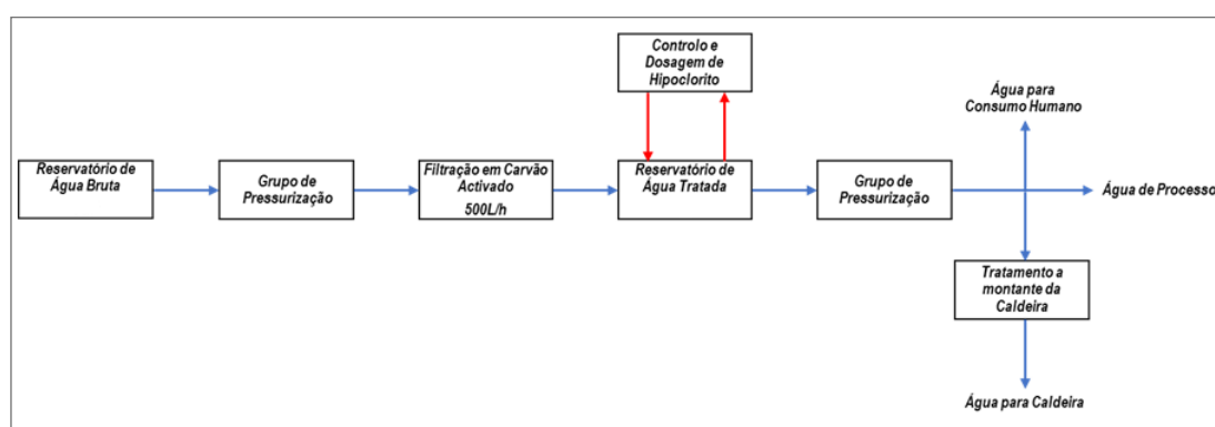
Figura III.24 – Esquema do tratamento da água do furo
