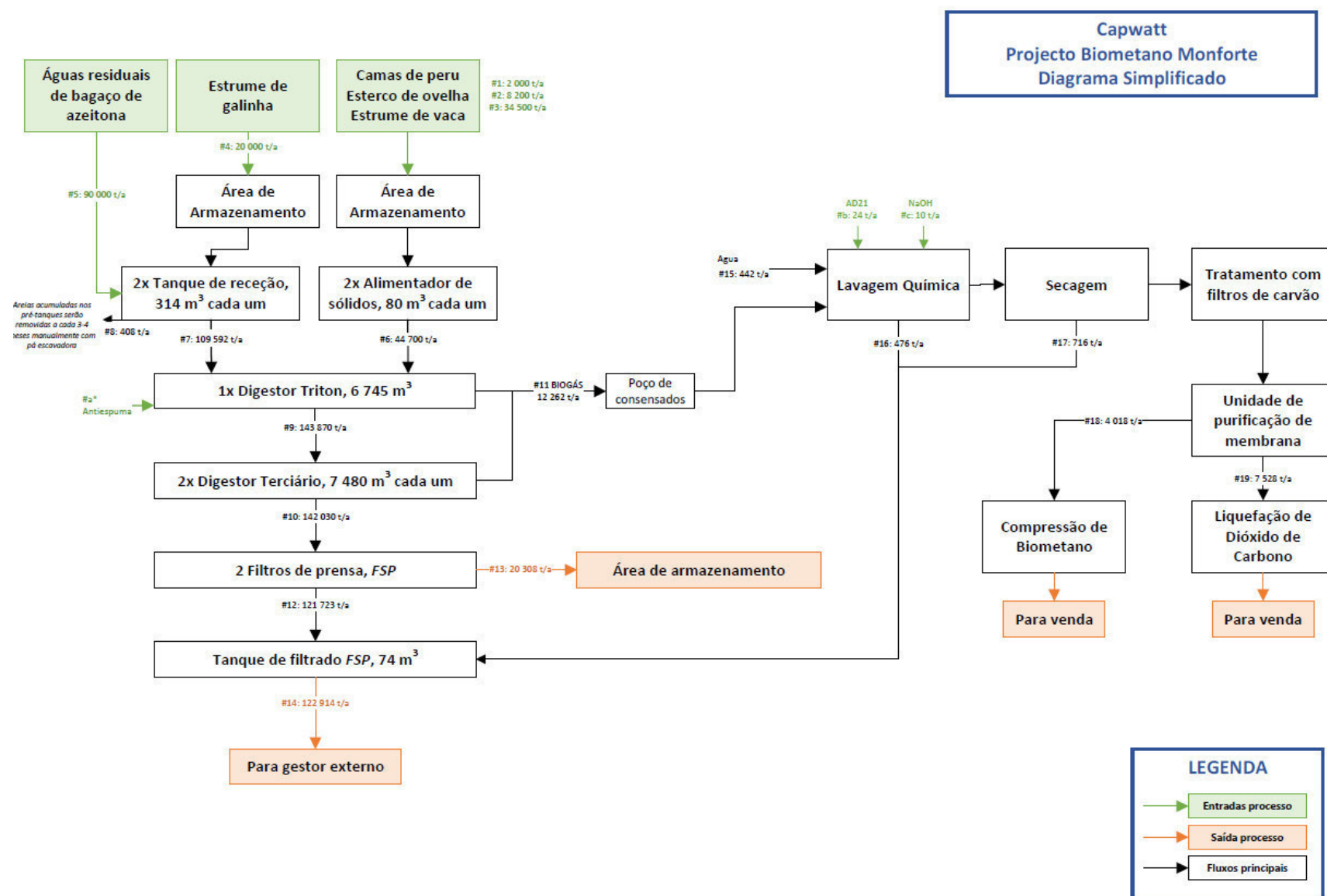
Figura III.27 – Balanços de massa da IPBB Monforte
