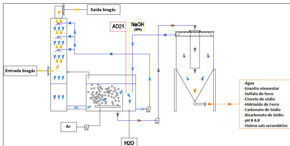
Figura III.18 – Equipamento de lavagem de biogás
