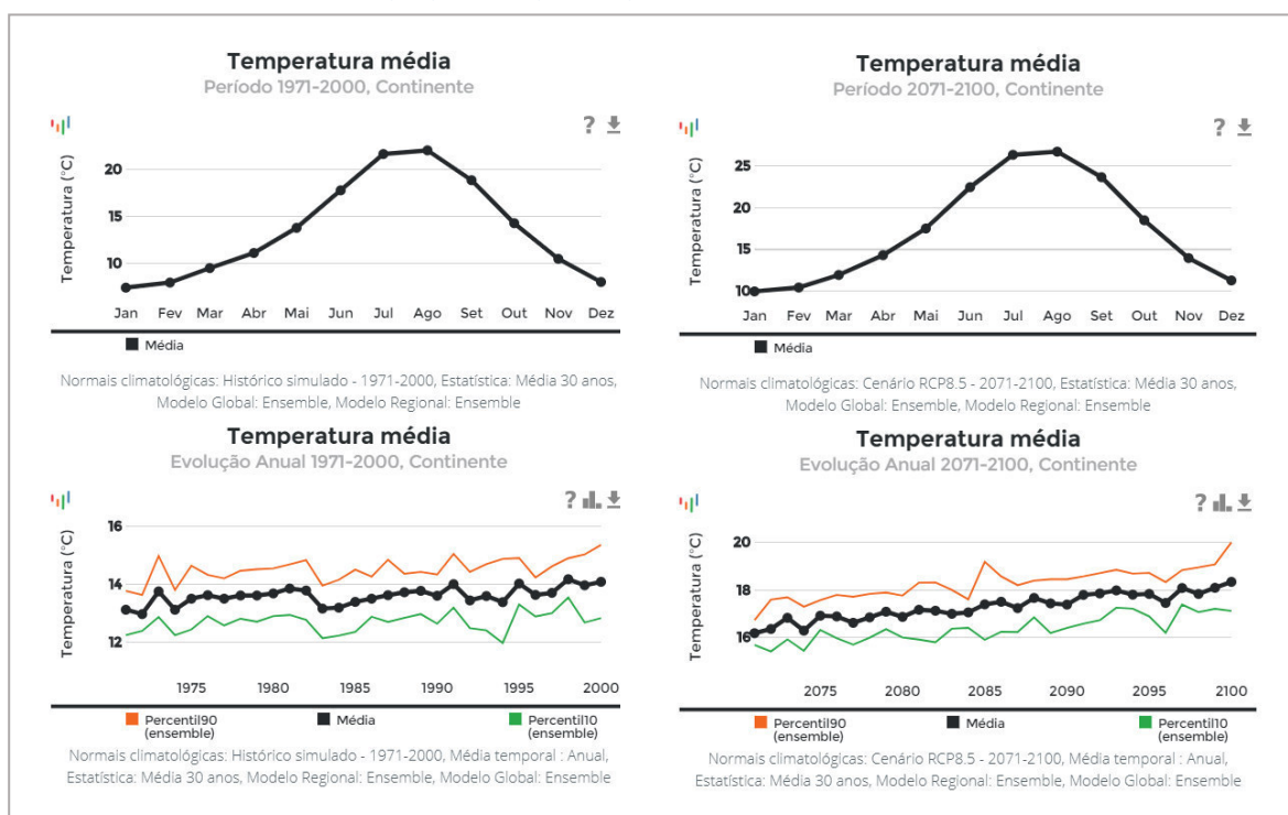
Figura IV.11 – Evolução da temperatura média no Continente entre 1971 e 2000 e anomalia projectada para o período de 2071-2100
