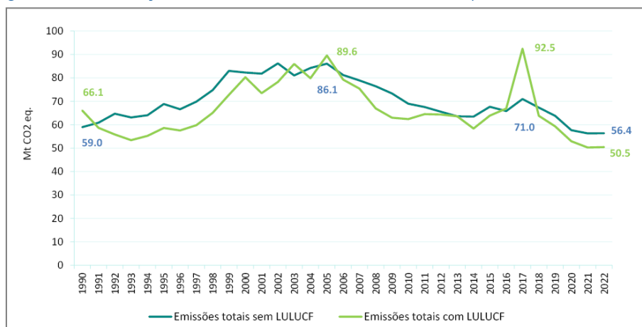
Figura IV.8 – Evolução das Emissões Nacionais de GEE no período 1990-2022
