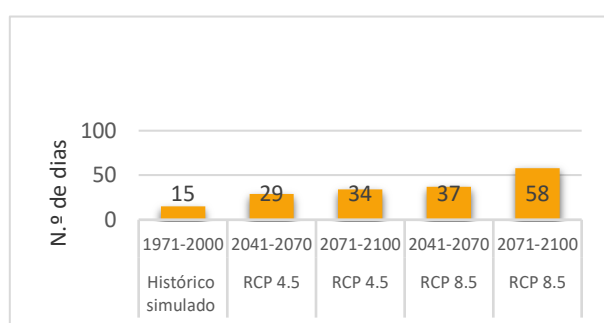
Figura IV.16 – Dias consecutivos muito quentes ( T \geq 35^{\circ}\text{C} ) – Alto Alentejo
