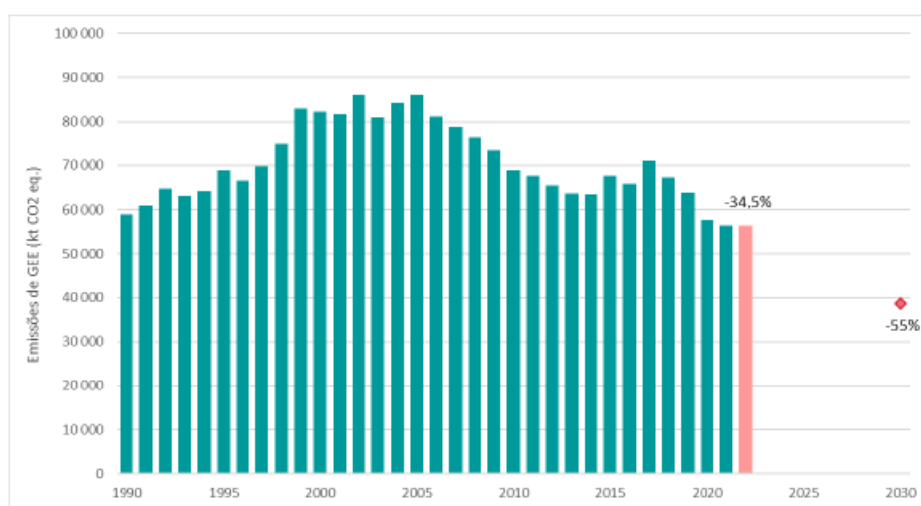
Figura IV.9 – Evolução das emissões nacionais de GEE (sem LULUCF) e evidência de cumprimento face às metas definidas no PNAC 2020 e PNEC 2030
