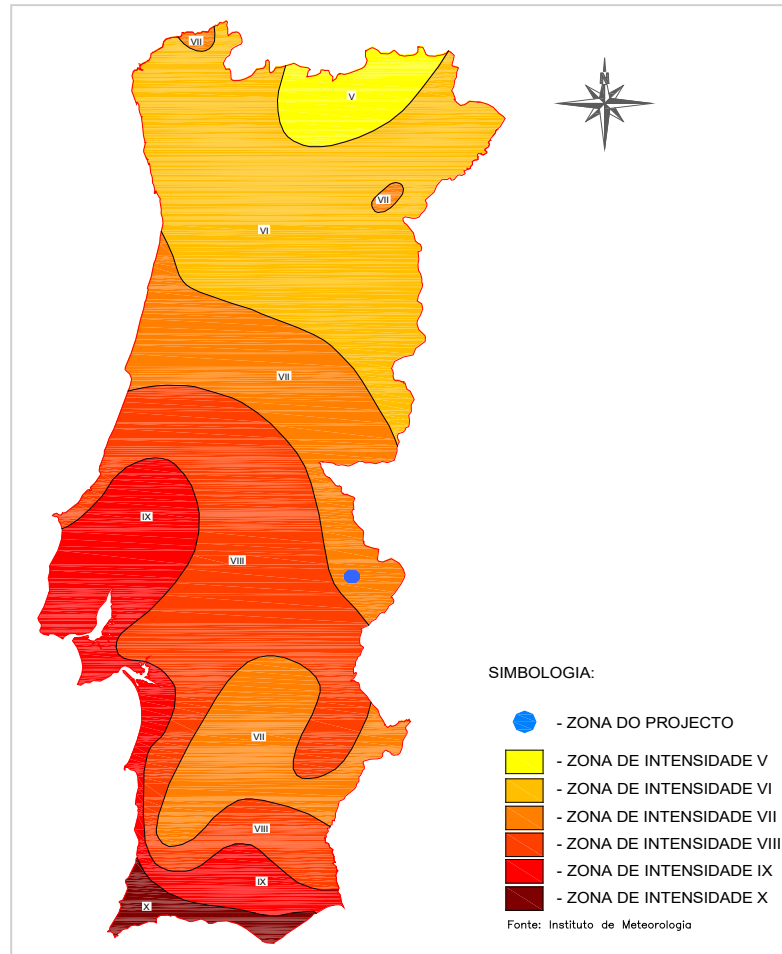
Figura IV.27 – Carta de Isossistas de Intensidades Máximas de Portugal Continental
