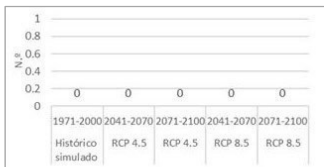
Figura IV.22 – Projecção do n.º de dias com ventos muito fortes ( \text{veloc.} > 39 \text{ km/h} ) Alto Alentejo
