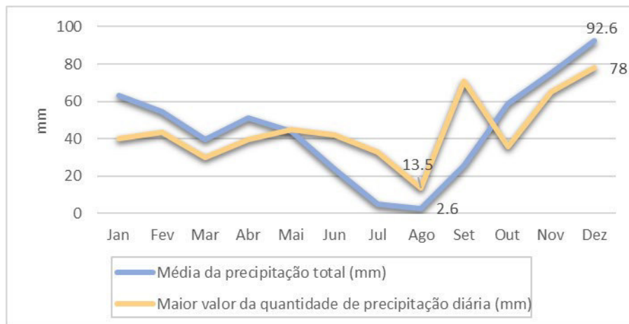
Figura IV.3 – Normais climatológicas dos valores de precipitação total e de precipitação máxima diária registados na Estação Meteorológica de Elvas, no período 1971-2000
