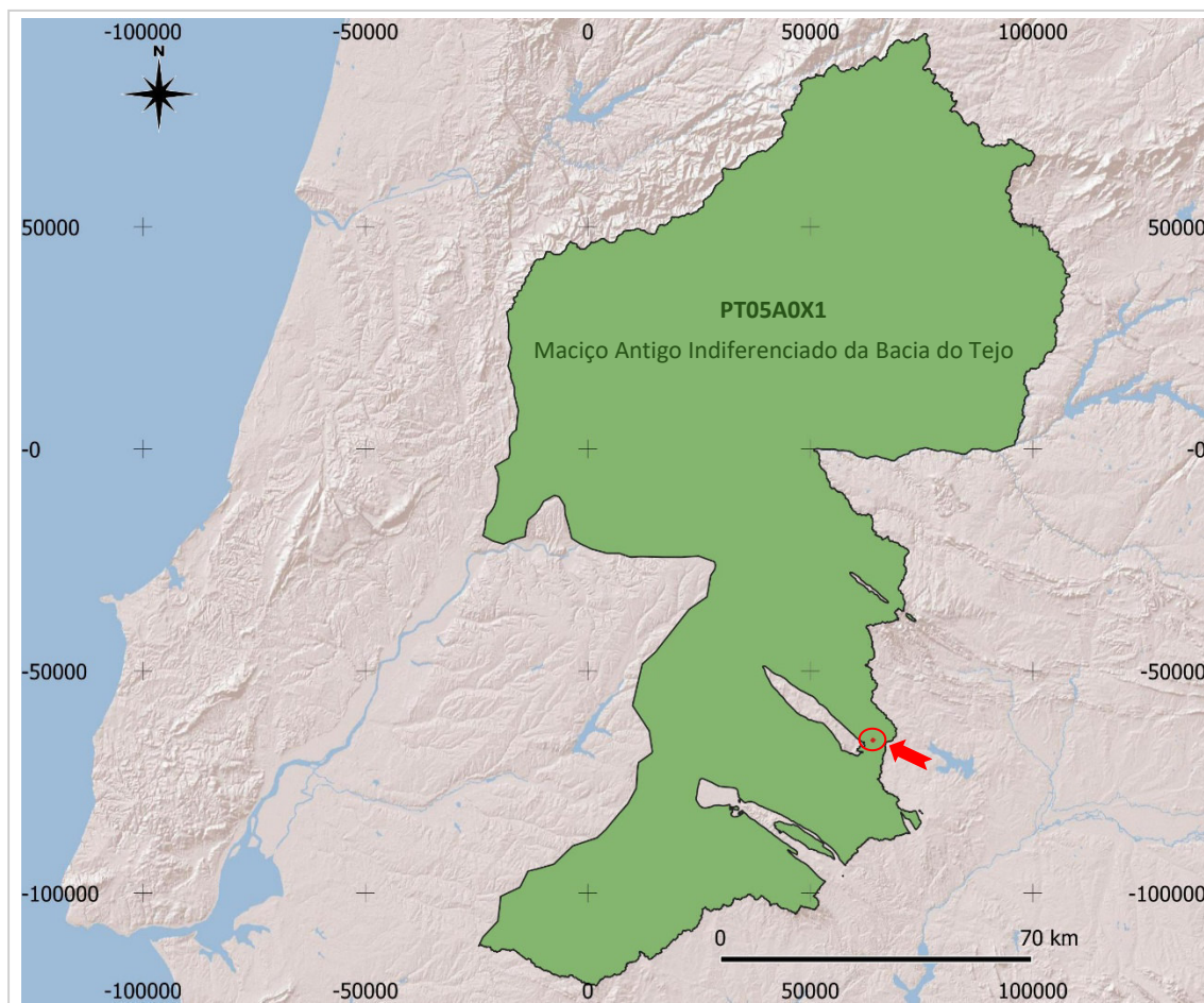
Figura IV.35 – Maciço Antigo Indiferenciado da Bacia do Tejo
