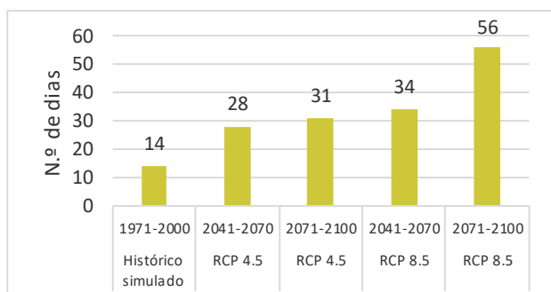
Figura IV.18 – Noites tropicais ( T > 20^{\circ}\text{C} ) Alto Alentejo
