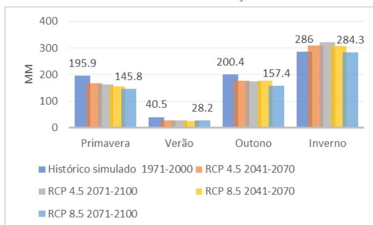
Figura IV.15 – Projecções da precipitação média anual por estação do ano – Alto Alentejo
