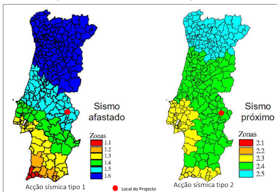
Figura IV.28 – Zonas sísmicas de Portugal Continental
