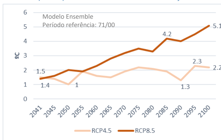
Figura IV.12 – Projecção da anomalia da temperatura máxima média anual para o período 2041 a 2100 – Alto Alentejo
