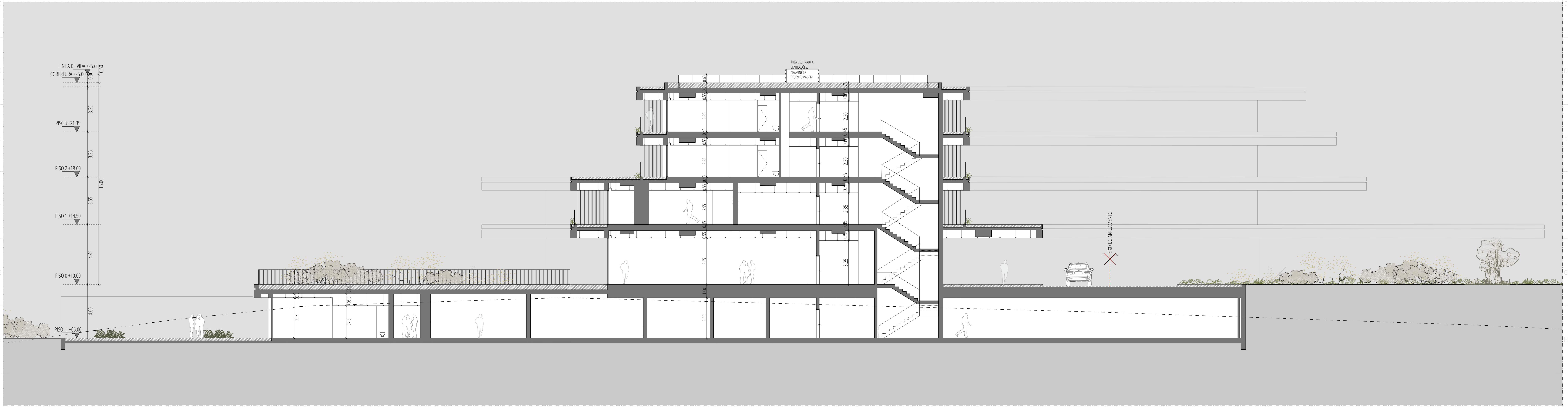
CORTE AA'
