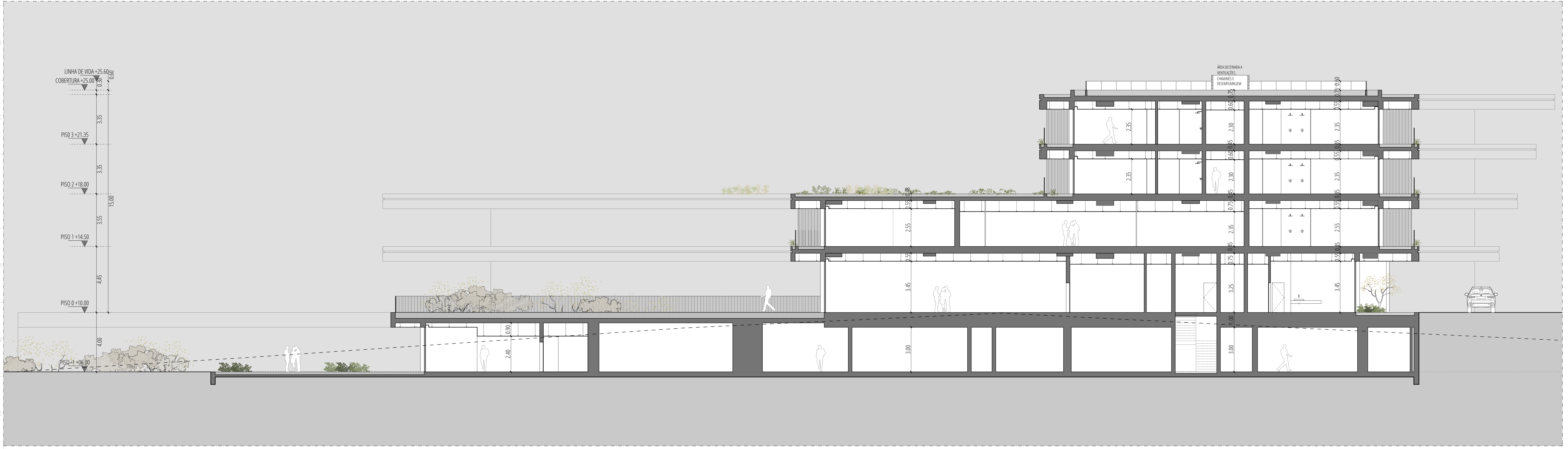
CORTE BB'
