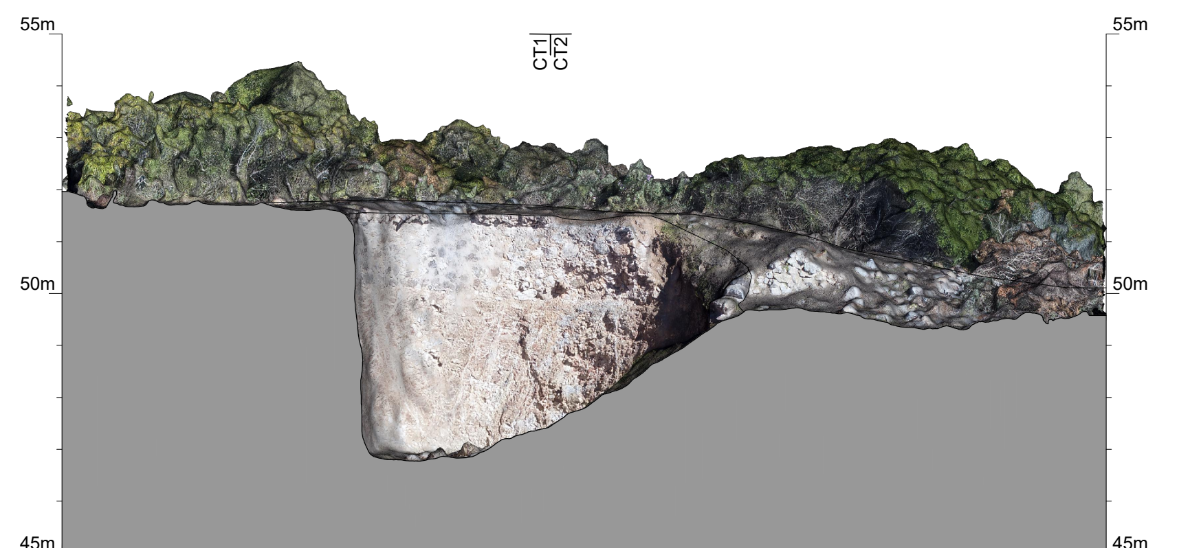
CORTE LONGITUDINAL 2
