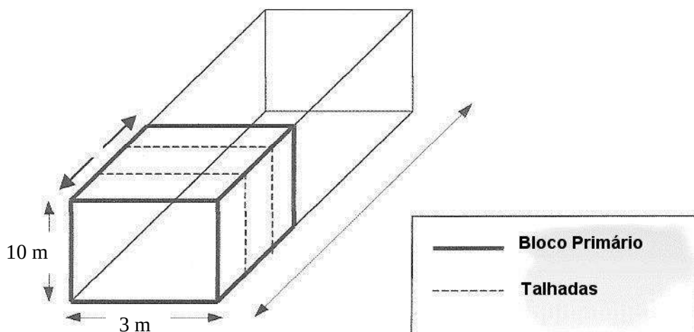
Figura 4 – Representação da individualização da bancada. Bloco primário e talhadas.
