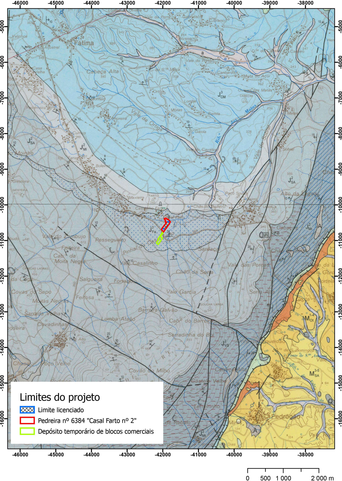
Figura 3 - Mapa geológico da envolvente à área da Área do Projeto (pedreira nº 6384 "Casal Farto nº 2"). Extrato da folha 27-A da Carta Geológica de Portugal à escala 1/50000, do ex. IGM (versão de 2000).
