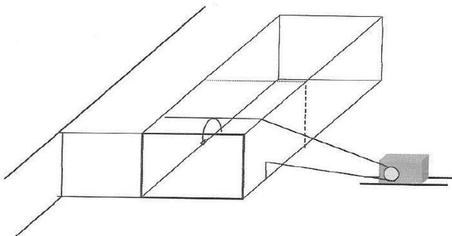
Figura 6 – Esquema de corte de uma fatia e direção de derrube.
